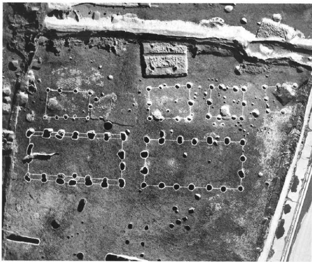
古代宮衛跡の掘立柱 建物跡群
