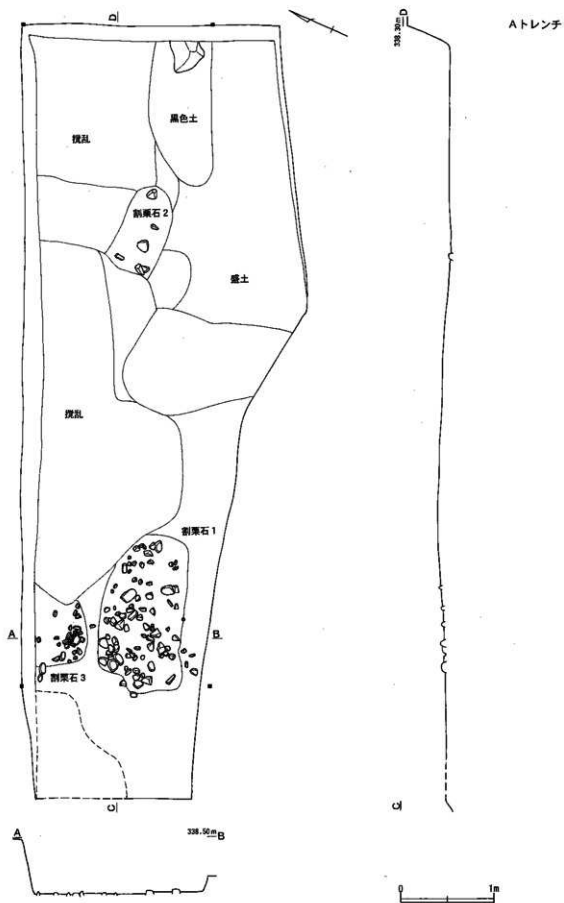
図6 本丸Aトレンチ平面図 (1:40)
