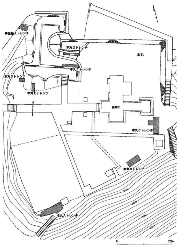
図5 本丸・帯曲輪トレンチ位置図 (1:400)
