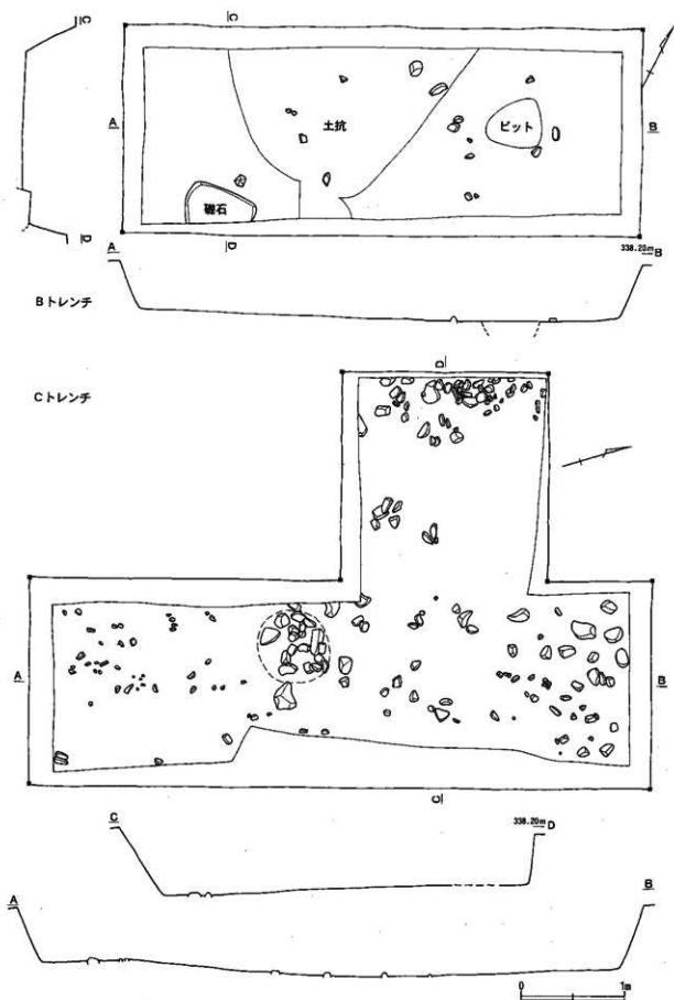
図7 本丸B・Cトレンチ平面図 (1:40)
