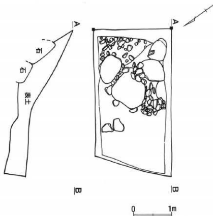
図10 帯曲輪Aトレンチ平面図 (1:50)
