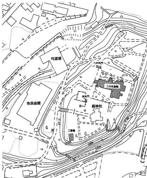
図19 確認遺構位置図 (1:2000)
