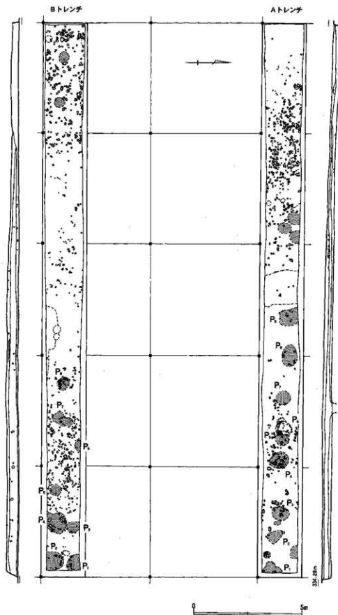
図12 二の丸A・Bトレンチ平面図 (1:120)
