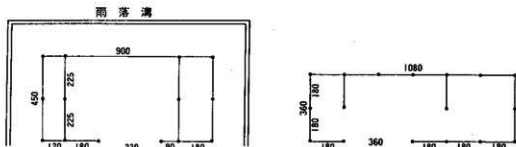
図3 南中門(左)及び駕籠部屋(右)規模模式図(1:200)単位はcm
