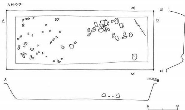
図18 三の丸Aトレンチ平面図 (1:40)
