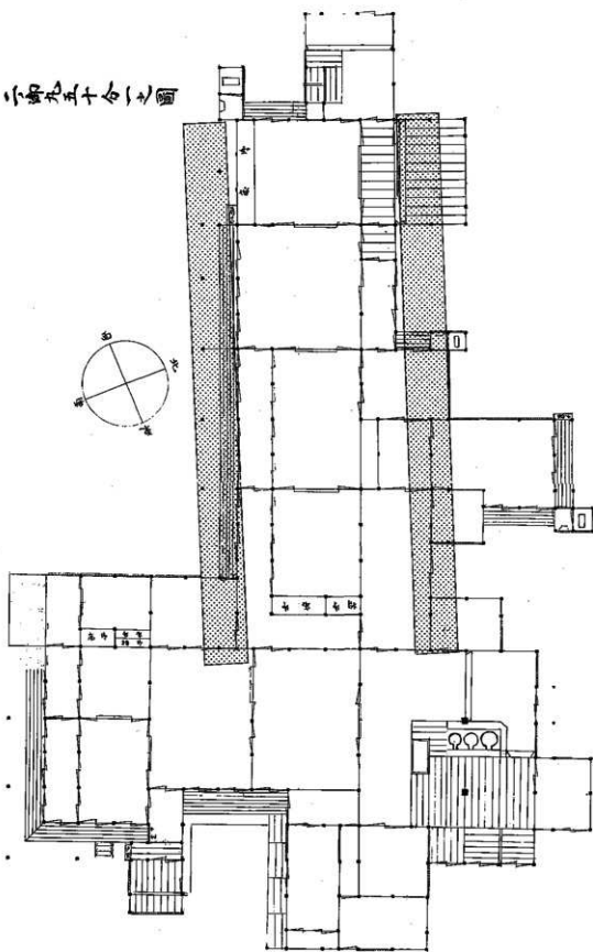
図13 二の丸御座敷取図及びトレンチ部定封圖 (1:200)
