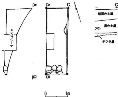
図8 本丸D・Eトレンチ平面図 (1:50)
