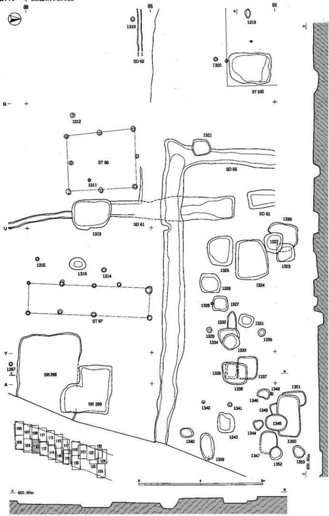
図版110 中世遺構実測図
