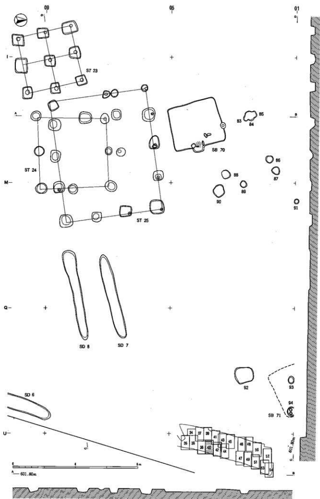
图版40 古代遺構実測図
