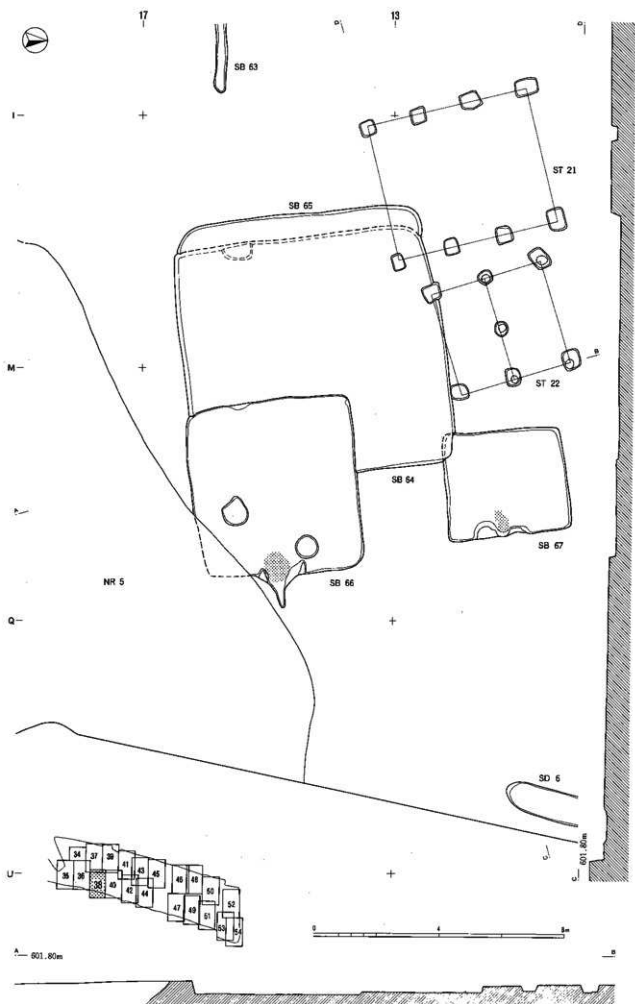
图版38 古代遺構実測図
