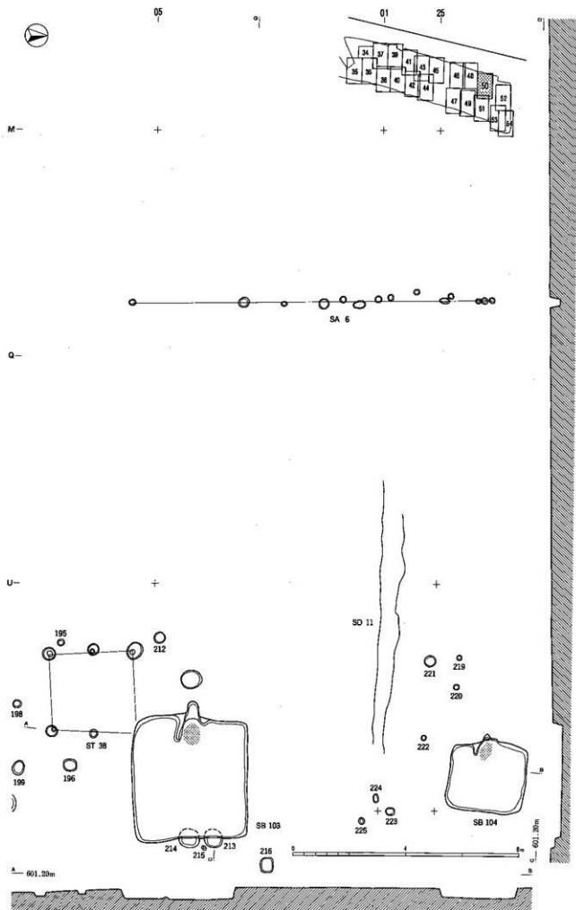
图版50 古代遺構実測図
