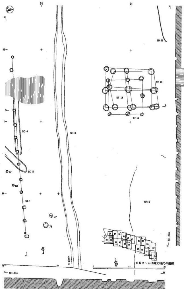
図版36 古代遺構実測図
