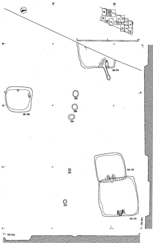
图版70 古代遺構実測図
