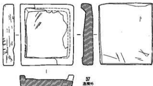
37 透輝石
