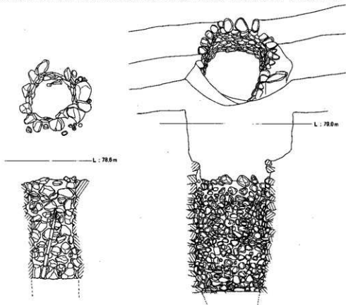
図18 SE811・SE812実測図(1/40)
