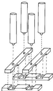
図6 SE011構造模式図(鈴木景二氏作成)
