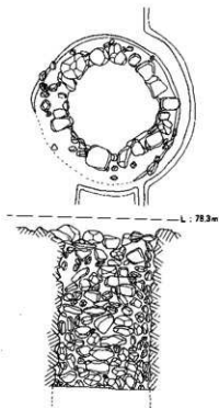
図17 SK711実測図(1/40)
