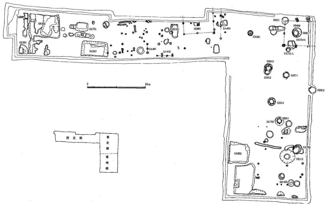
图4 遺構配置図 (D~H期)
