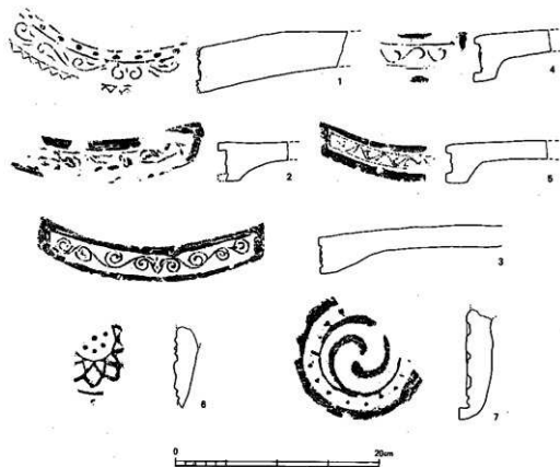
第13图 軒瓦
