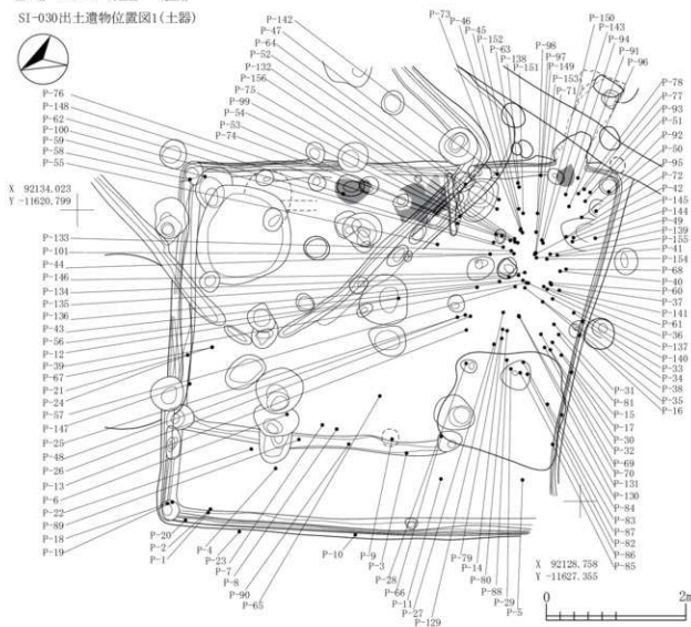
図 2-123 竪穴住居跡 -122
