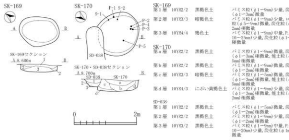
図 2-322 土坑-35
