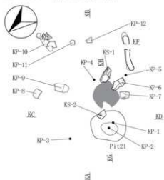
SI-010bカマド出土遺物位置図
