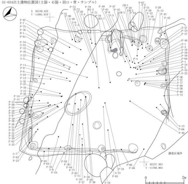
SI-034出土物位置図(土器・石器・羽口・骨・サンプル)
