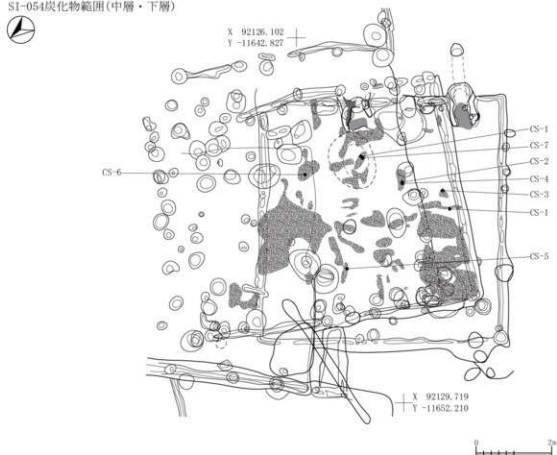
SI-054炭化物範囲(中層・下層)
