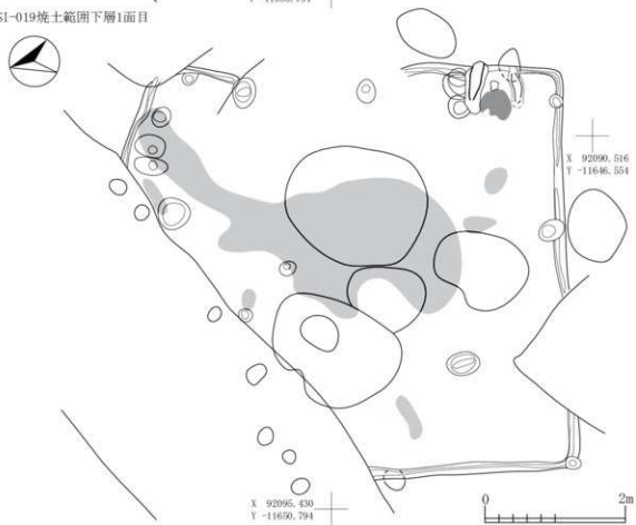
図 2-76 竪穴住居跡 -75
