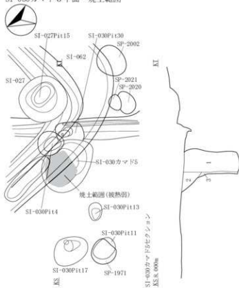
SI-030カマド5平面・焼土範囲
