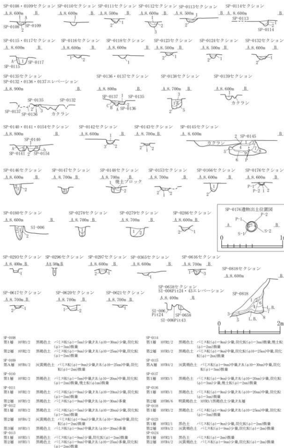
図 2-475 ビット -63
