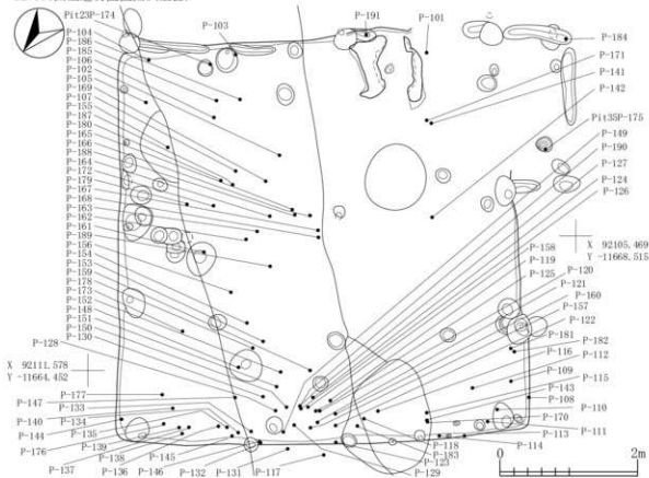
SI-006出土遺物位置圖2(土器)
