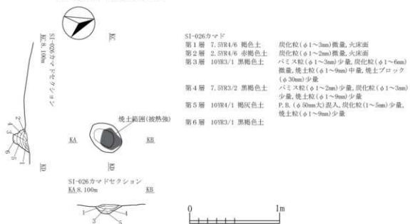
図 2-107 竪穴住居跡-106
