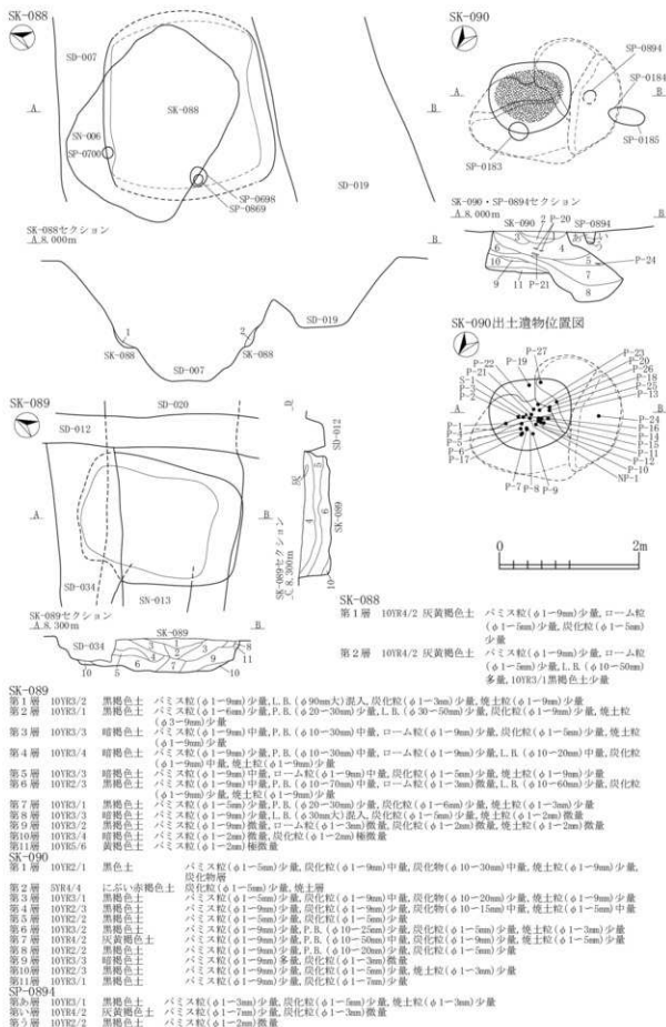
図 2-307 土坑-20
