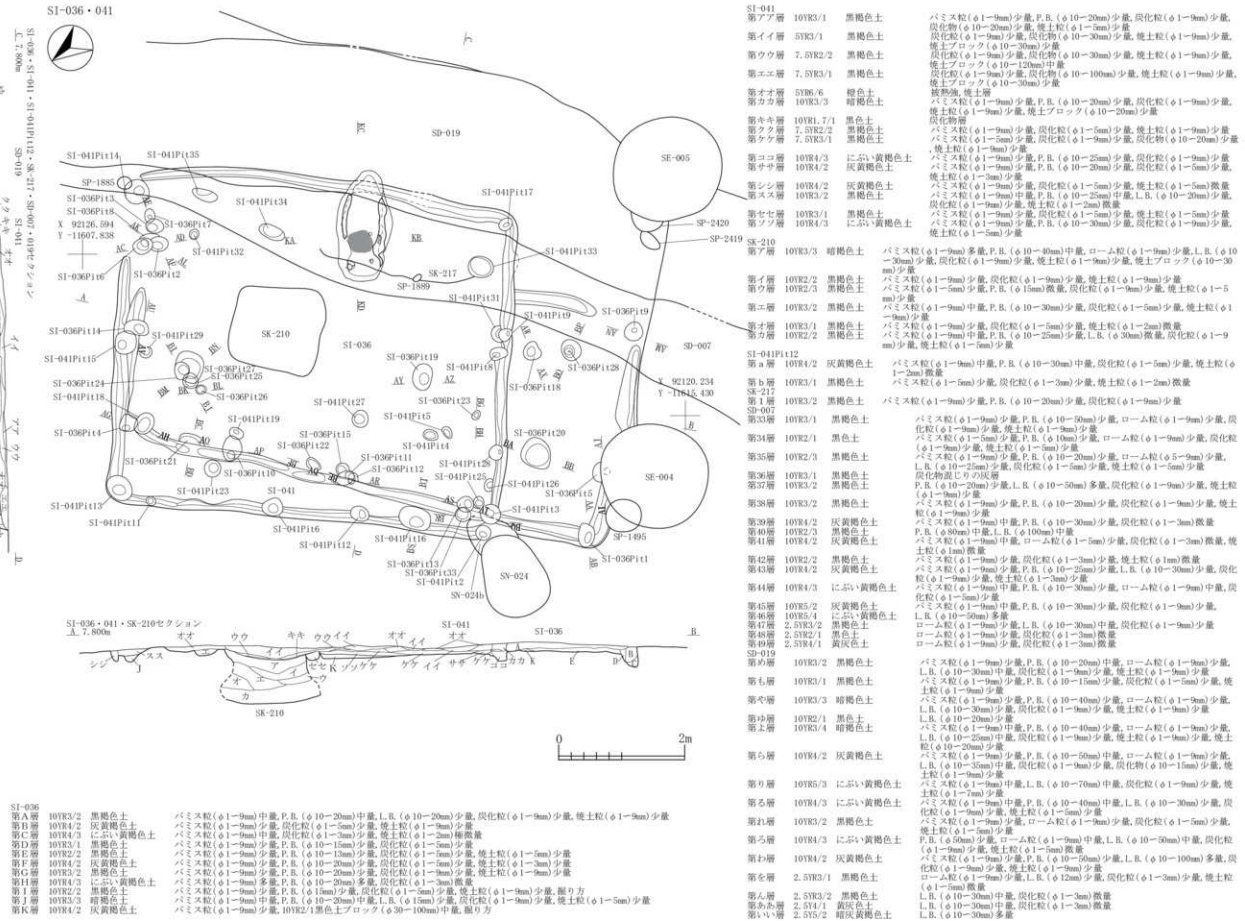
図 2-164 竪穴住居跡 -163 - 199 - 200 -
