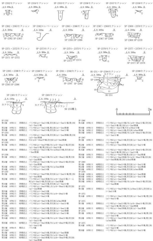
図 2-430 ビット -18
