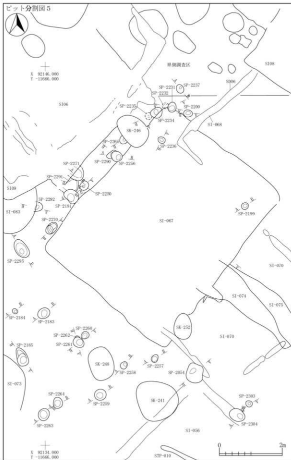
図 2-423 ビット -11
