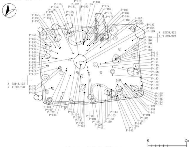
图 2-87 竖穴住居跡-86
