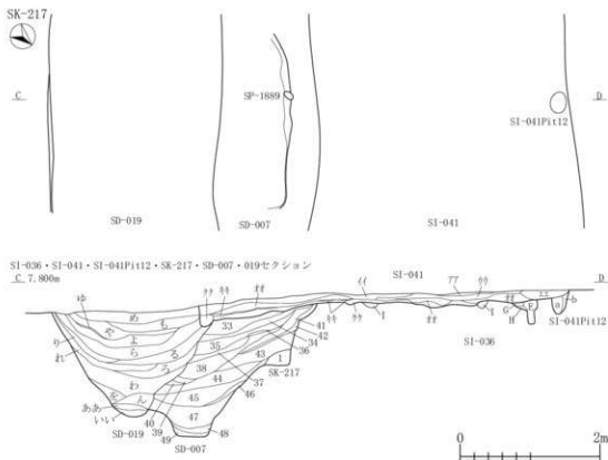
図 2-333 土坑-46
