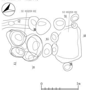
SI-052SN-01・02掘り方
