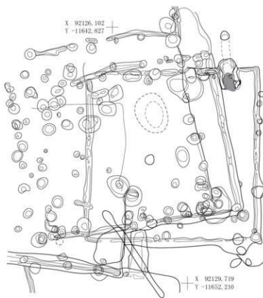
SI-054掘り方
