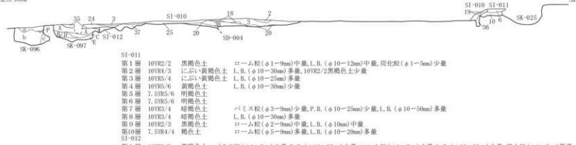
SK-010・011・012・SK-096・097セクション・SD-004・SK-025エレベーション 5.8, 900m
