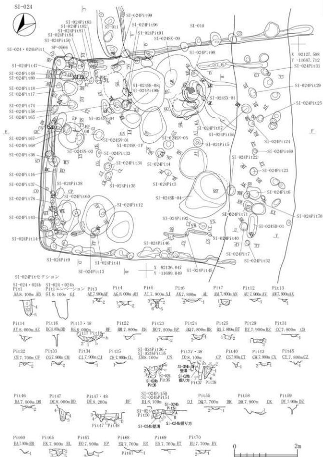
図 2-93 竪穴住居跡 - 92
