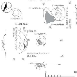
SI-024SN-01・03・04炭化物・焼土範囲1目面
