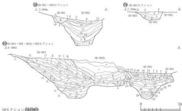
SDセクション 58 59 60
