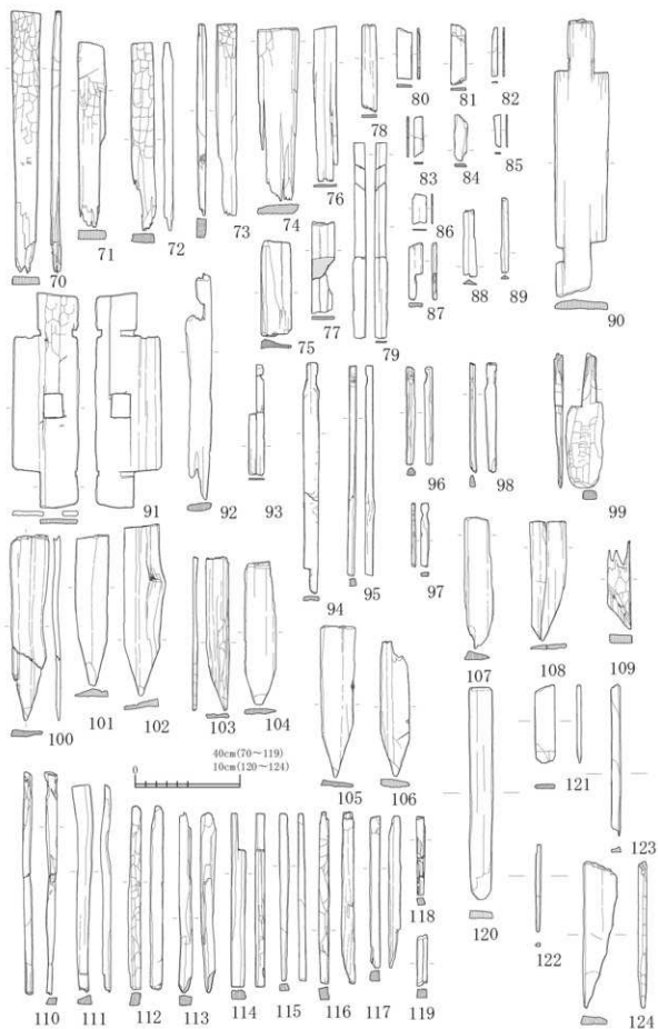
図 W-1-6 A区 SF-01木組遺構
