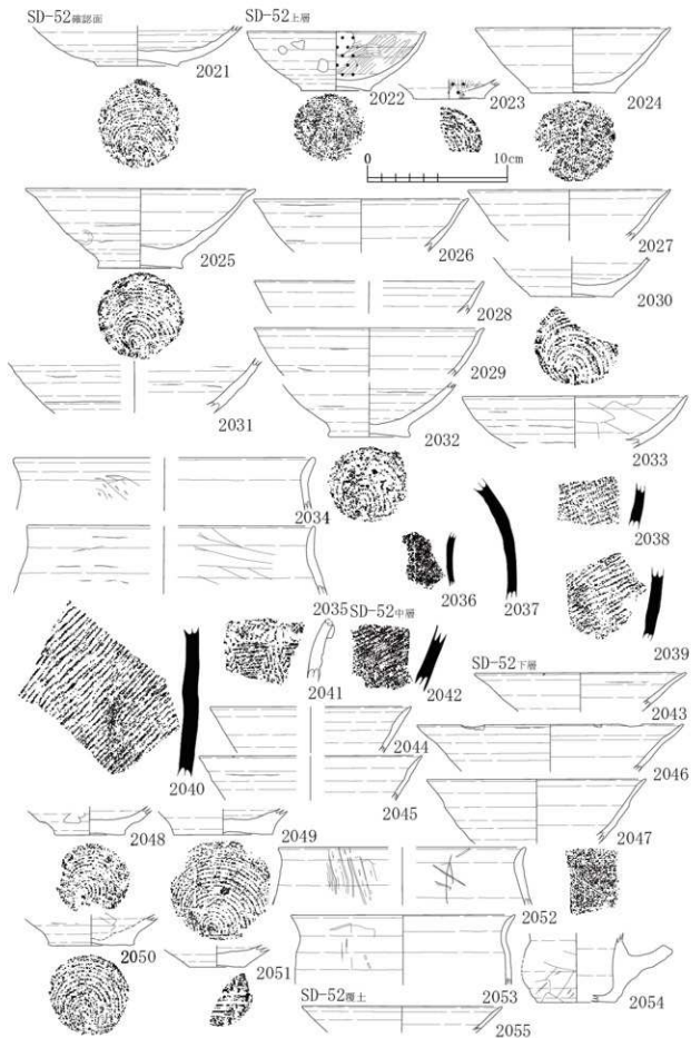
図 P-1-078 丘陵地部分溝跡
