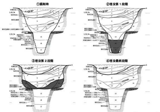
第16図 SK-101埋没過程変遷図 (S=1/50)
