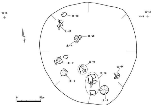
第15図 SK-101上層上位 遺物出土状況図 (S=1/20)
