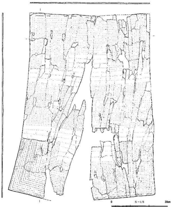
第27図 SK-101出土木製盾
