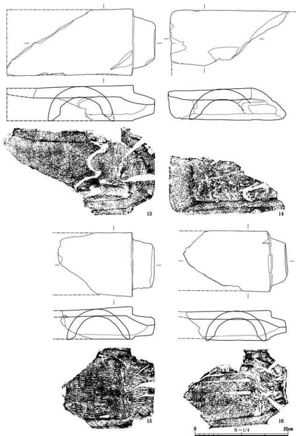
第25圖 SK-01出土瓦3
