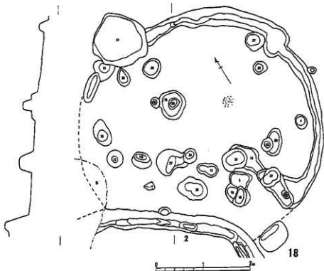
第15图 17·18号住居址
