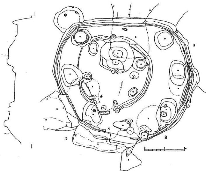
第12图 8号住居址
