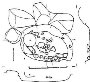
第18図 11号住居址, 配石墓, 土壌802号
