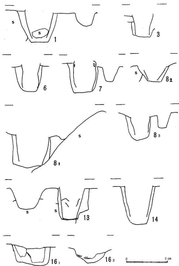
第43圖 埋壙埋設狀況
