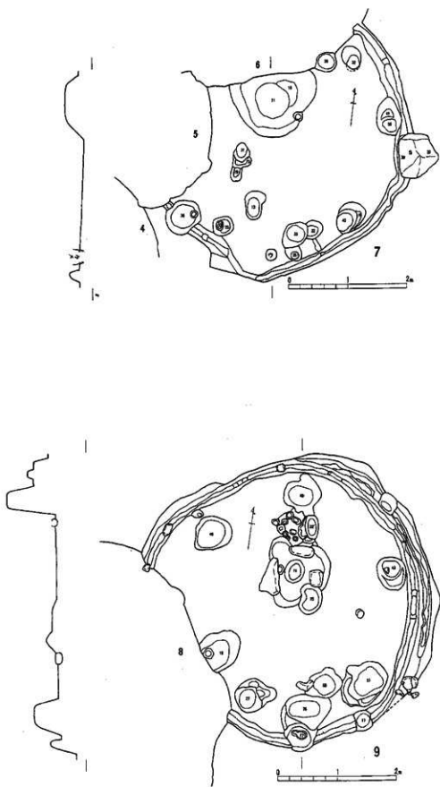
第11图 7·9号住居址
