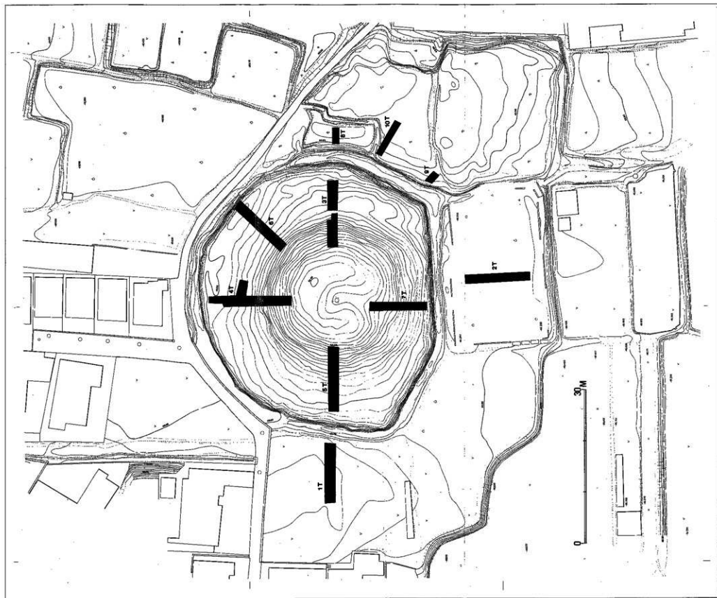
图3 トレンチ位置図
