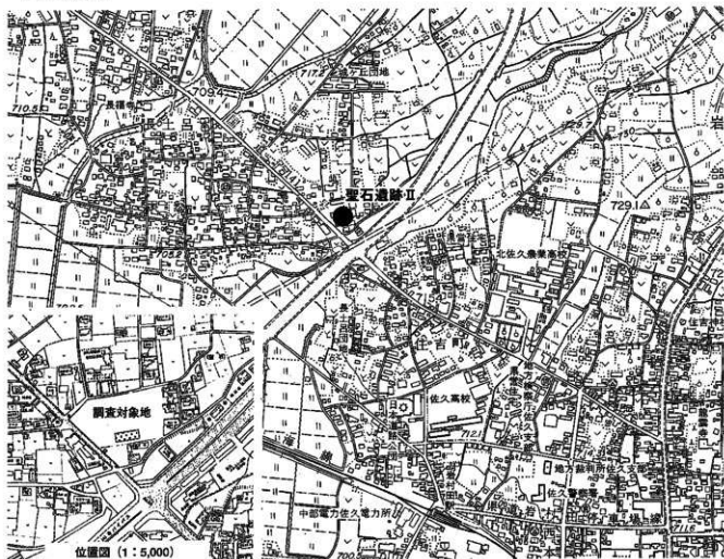
第1図 聖石遺跡Ⅱ 位置図 (1:10,000)
