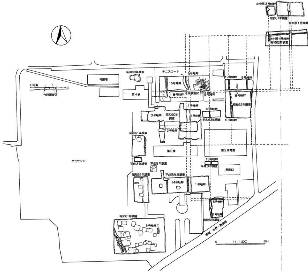
第17図 馬口遺跡・北中原遺跡雑群位置図
