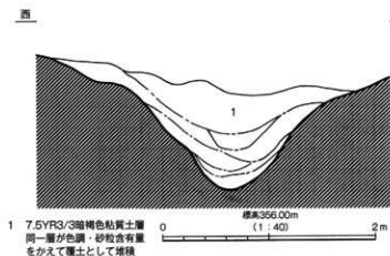
第7図 1号溝跡土層断面図 (トレンチ北壁部)
