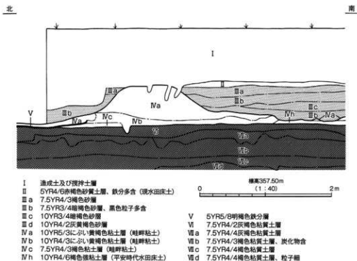
第15図 8号畦畔土層断面図(トレンチ東壁面)
