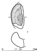
第8図 1号溝跡出土石器 実測図
