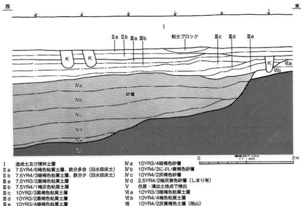
第9図 トレンチ西端旧河道部分土層断面図 (トレンチ北壁側)
