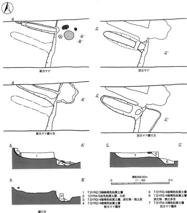
第5図 1号住居跡カマド実測図
