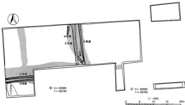
第11図 テニスコート地点 平安時代水田面畦畔遺構実測図 (網点=平安時代水田面畦畔)
