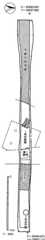
第3図 グラウンド地点トレンチ遺構全体図
