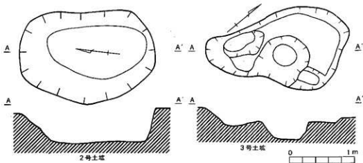
第7図 2・3号土坑実測図
