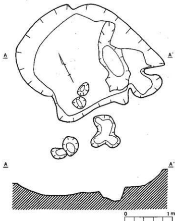
第6図 1号土壇実測図
