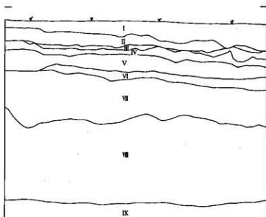
第13図 土層断面図（A-1グリッド北壁）
