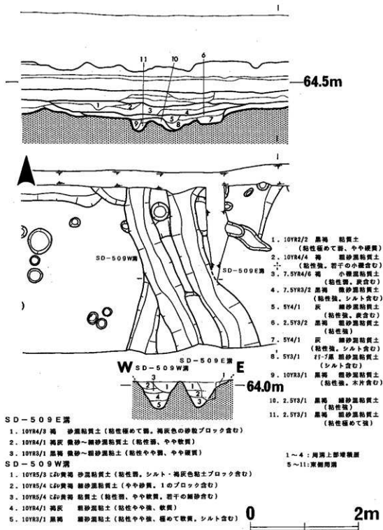
図6 東端遺構群平面・土層図 (S=1/50)
