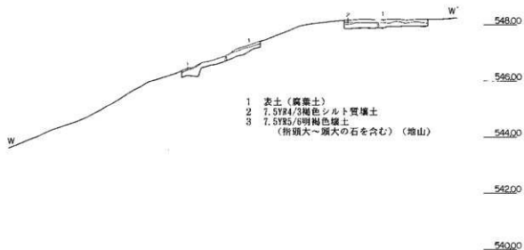
榛名山古墳実測図
