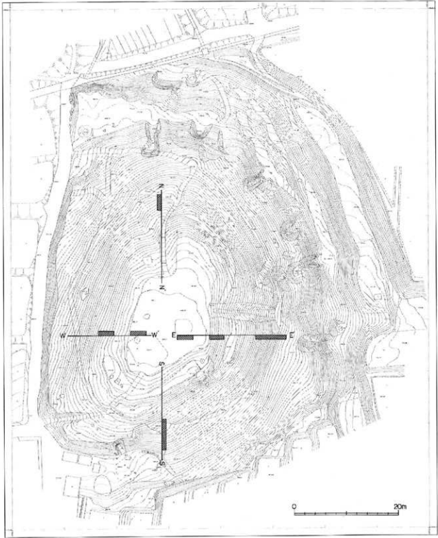
榛名山古墳地形図
