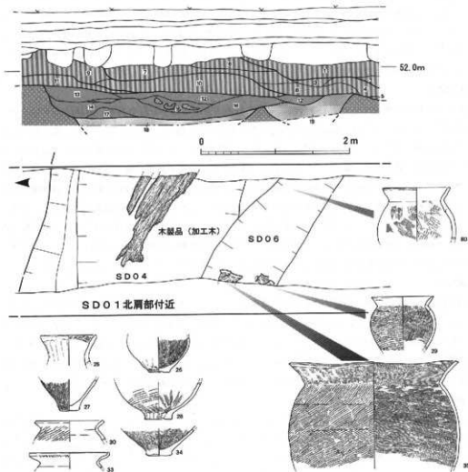
西トレンチ (南) 東壁 方形区画大溝SD01北肩部付近土層断面図
