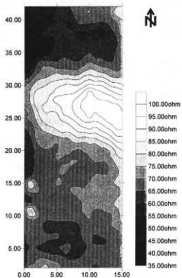
3 電気探査 平面図
