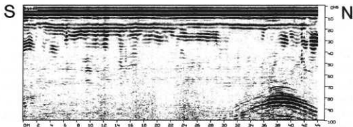
1 レーダー探査 断面図 X=7mライン
