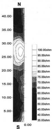
2 電気探査 断面図 X=7mライン (左辺が地表面)
