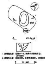
第32図 D26号土坑実測図
