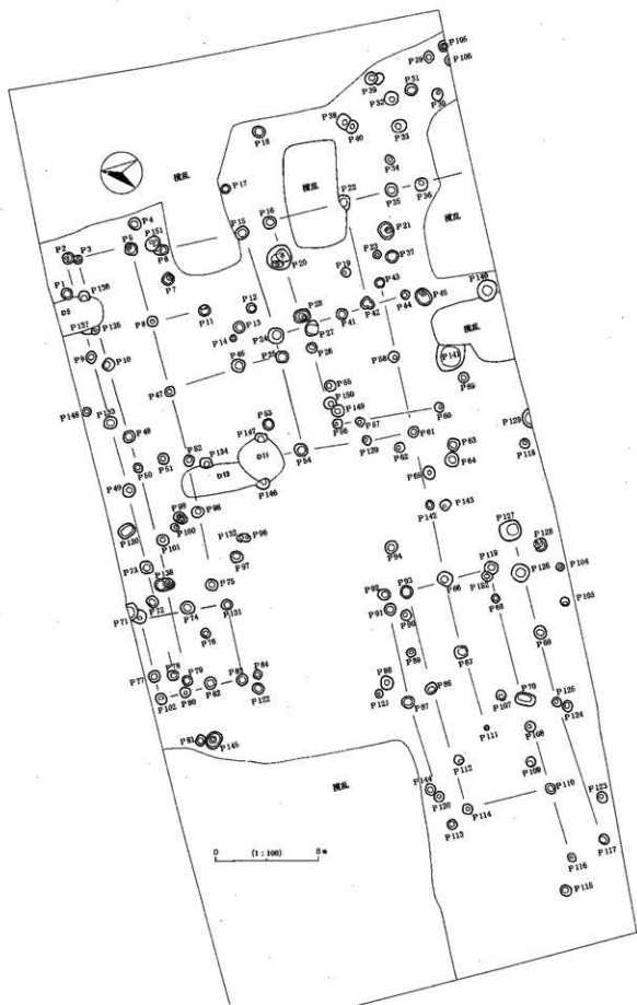
第40图 柱穴柱实测图
