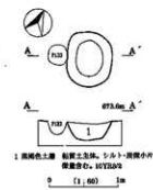
第36図 D30号土坑実測図
