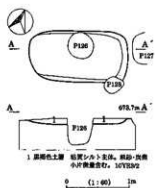
第26図 D20号土坑実測図
