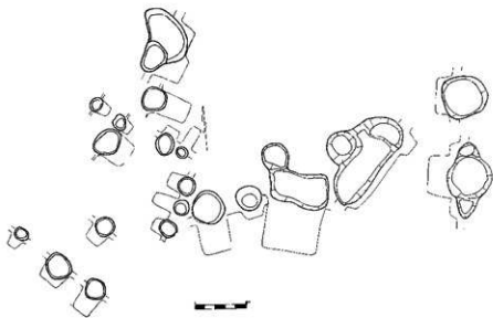
第8图 上墳实测图 (S=1/80)
