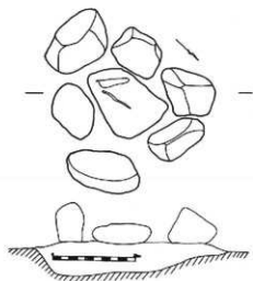
第68図 大城林配石3実測図(S=1/10)
