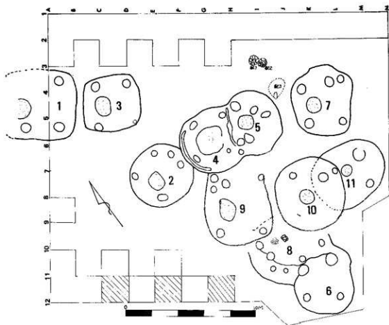
第78図 北方I遺構全体図 (S=1/200)
