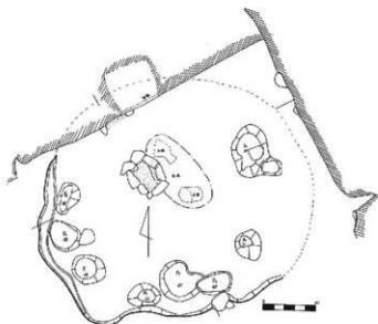
第11図 大城林第5号住居址実測図 (S=1/80)
