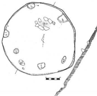
第13図 大城林第6号住居址実測図 (S=1/80)
