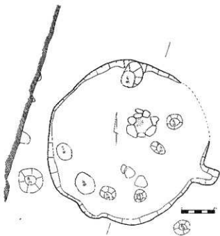
第29図 大城林第15号住居址実測図 (S=1/80)
