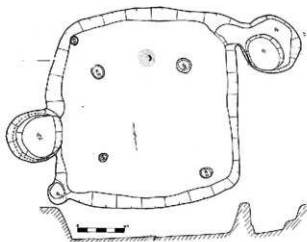
第4図 第2号住居址実測図(S=1/80)
