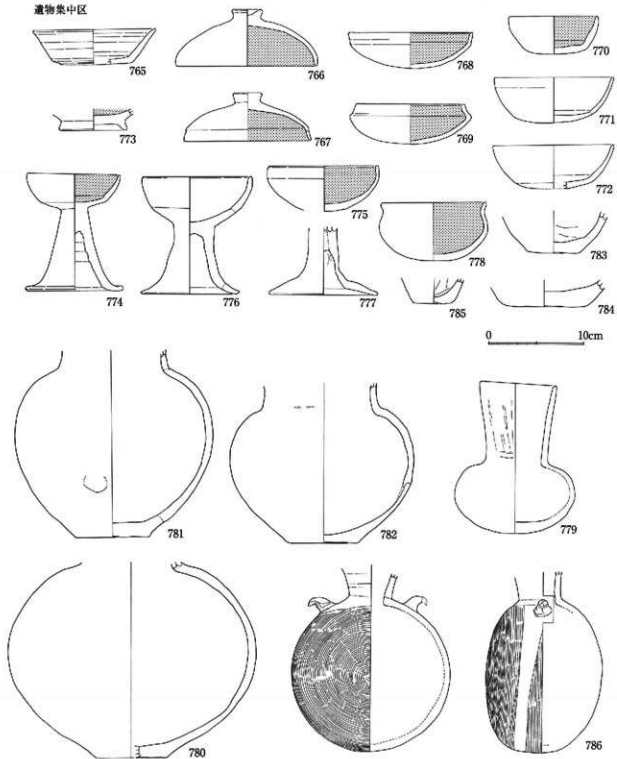
图47 平成6年度調査 遺物実測図③(1:4)
