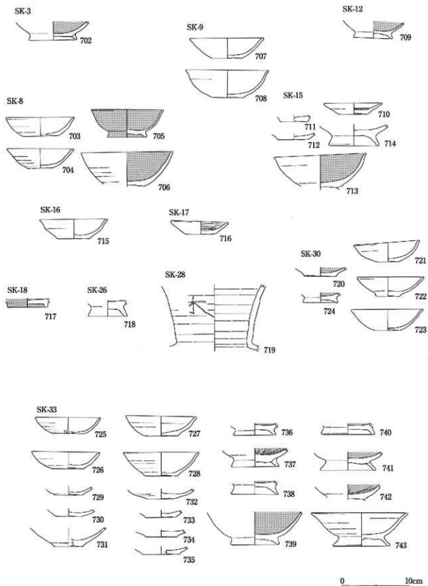
図45 平成6年度調査 遺物実測図② (1:4)
