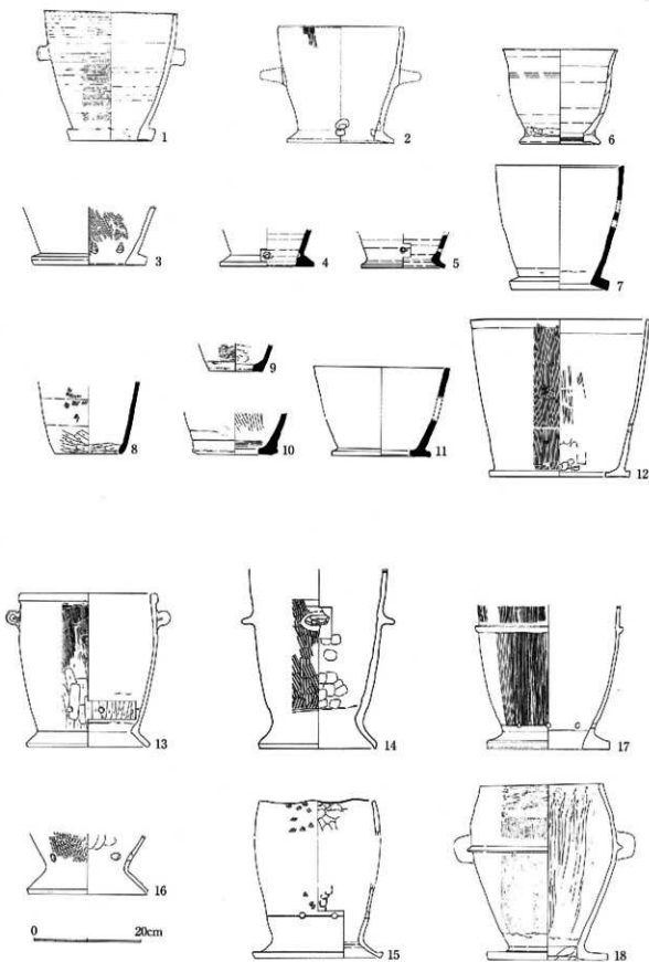
図15 長野県内出土の甕 集成図① (1:8)
