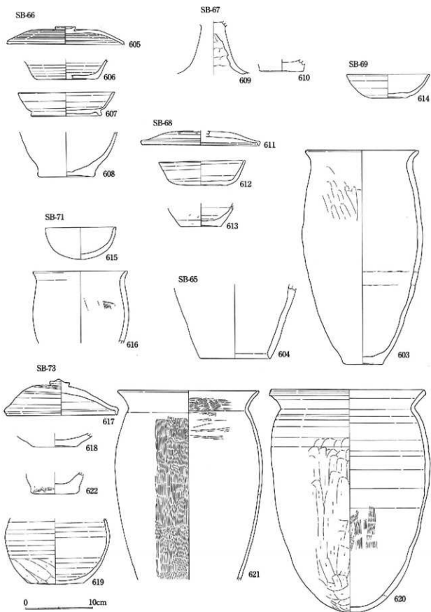
図42 平成6年度調査 遺物実測図⑧ (1:4)
