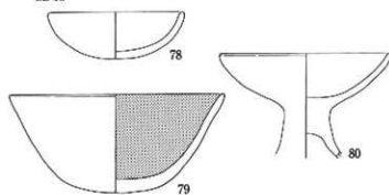
図18 平成6年度調査 遺物実測図② (1:4)
