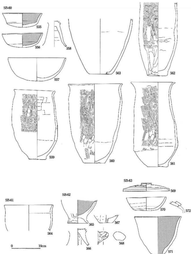
図39 平成6年度調査 遺物実測図② (1:4)
