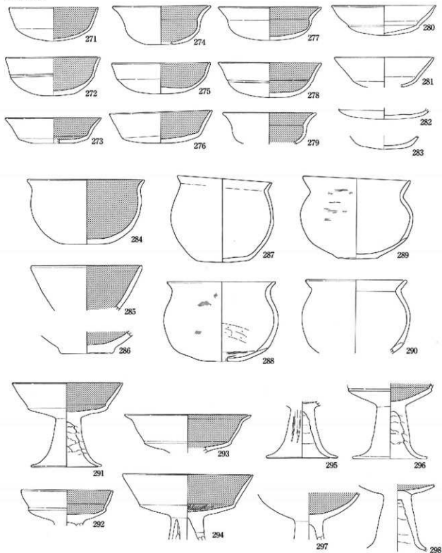
图28 平成6年度調査 遺物実測図② (1:4)
