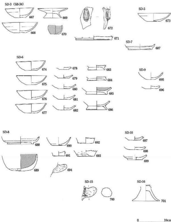
図44 平成6年度調査 遺物実測図② (1:4)
