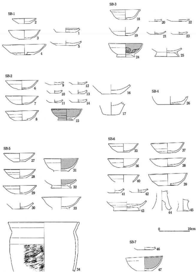
図17 平成6年度調査 遺物実測図① (1:4)
