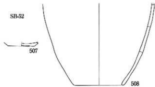
図36 平成6年度調査 遺物実測図② (1:4)
