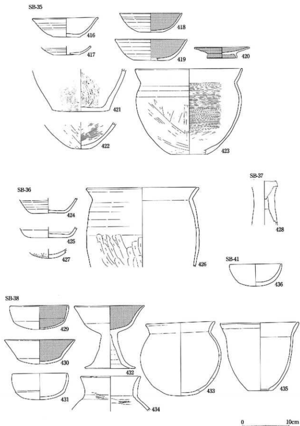
図33 平成6年度調査 遺物実測図⑦ (1:4)
