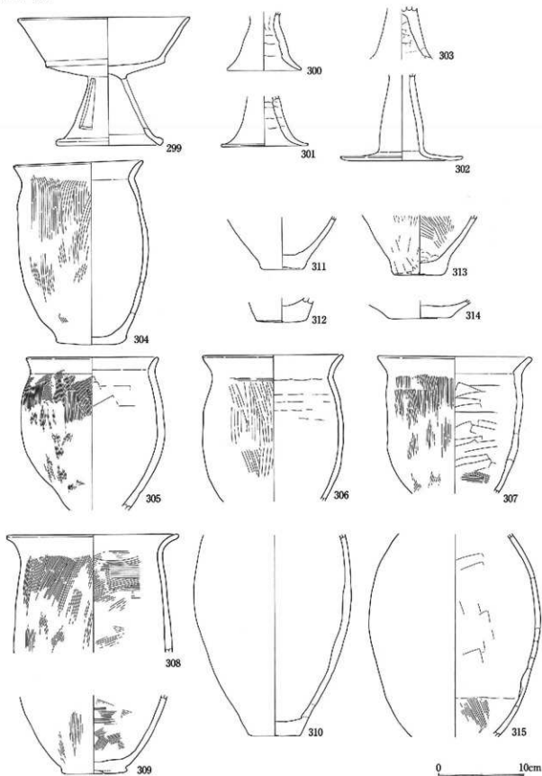
图29 平成6年度調査 遺物実測図⑬ (1:4)
