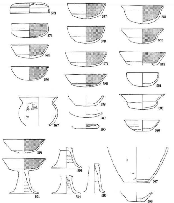
图40 平成6年度調査 遺物実測図⑧ (1:4)
