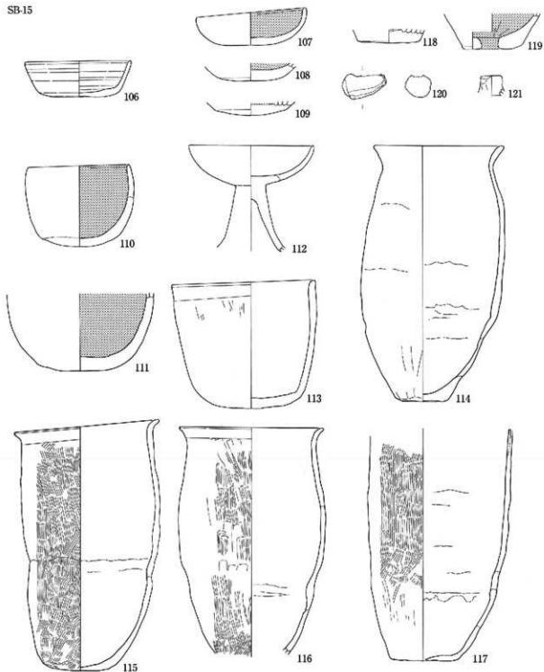
图20 平成6年度調査 遺物実測図④ (1:4)
