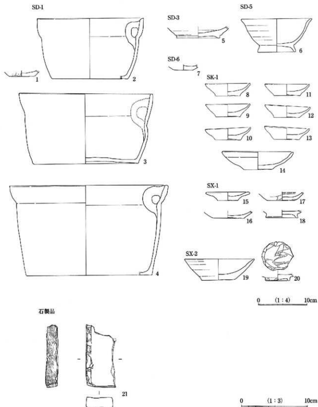
図52 平成7年度調査 遺物実測図 (1~20=1:4 21=1:3)
