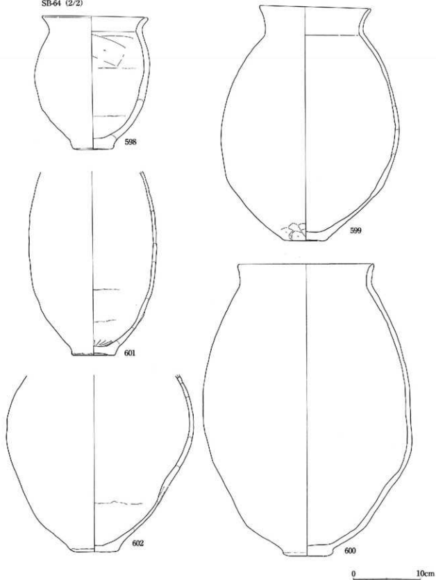
図41 平成6年度調査 遺物実測図② (1:4)
