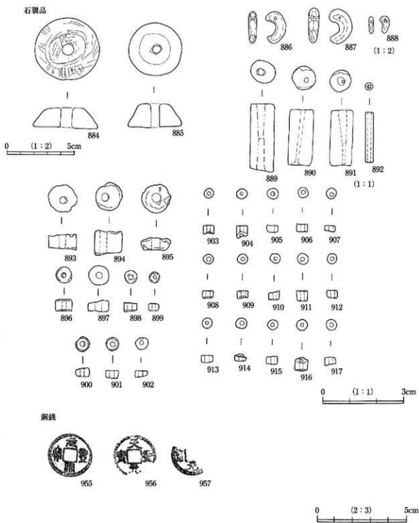
図51 平成6年度調査 遺物実測図⑤ (石製紡錘車・勾玉1:2 管玉・白玉1:1 銅銭2:3)
