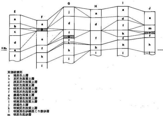
図11 柱状図 (S=1:80)
