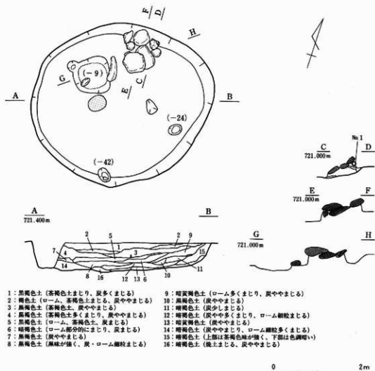
第51図 第8号住居址実測図 S=1/60
