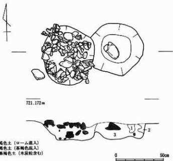
第100図 第4号集石炉実測図 S = 1/20
