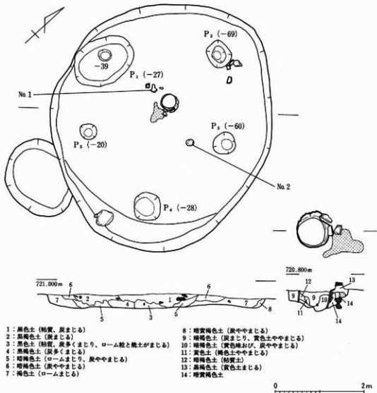
第12図 第3号住居址実測図 S=1/60 (炉:S=1/30)
