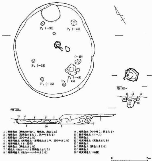
第85図 第14号住居址実測図 S=1/60 (炉: S=1/30)
