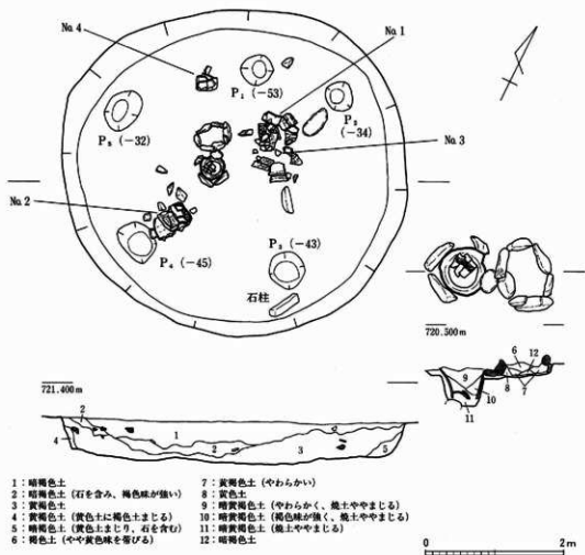
第33図 第6号住居址実測図 S=1/60 (炉: S=1/30)
