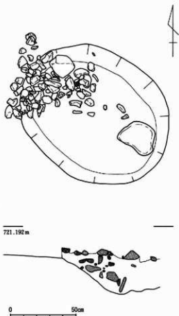
第98図 第1号集石炉実測図 S=1/20
