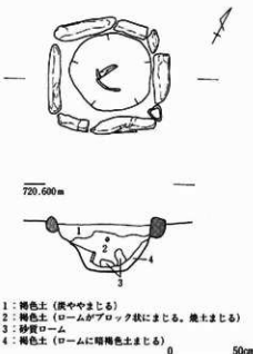
第65図 第11号住居址炉実測図 S=1/30
