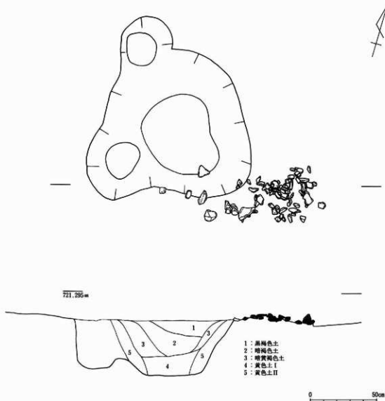
第107図 第9号集石炉実測図 S = 1/20
