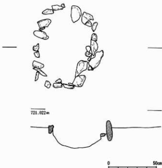
第113図 第17号集石炉実測図 S = 1/20
