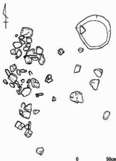
第97図 第2号集石実測図 S=1/30
