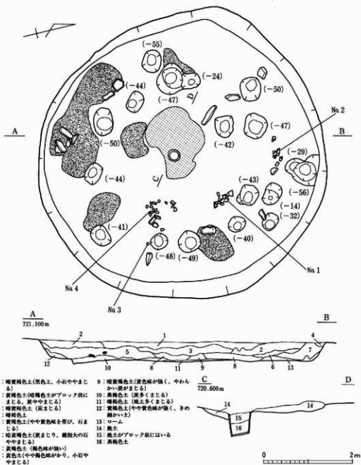
第55図 第9号住居址実測図 S=1/60 (炉: S=1/30)
