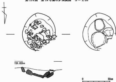
第115図 第20号集石炉実測図 S = 1/20
