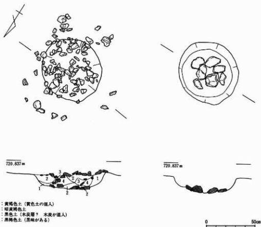
第114図 第19号集石炉実測図 S = 1/20
