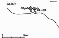
第108図 第10号集石炉実測図 S = 1/20
