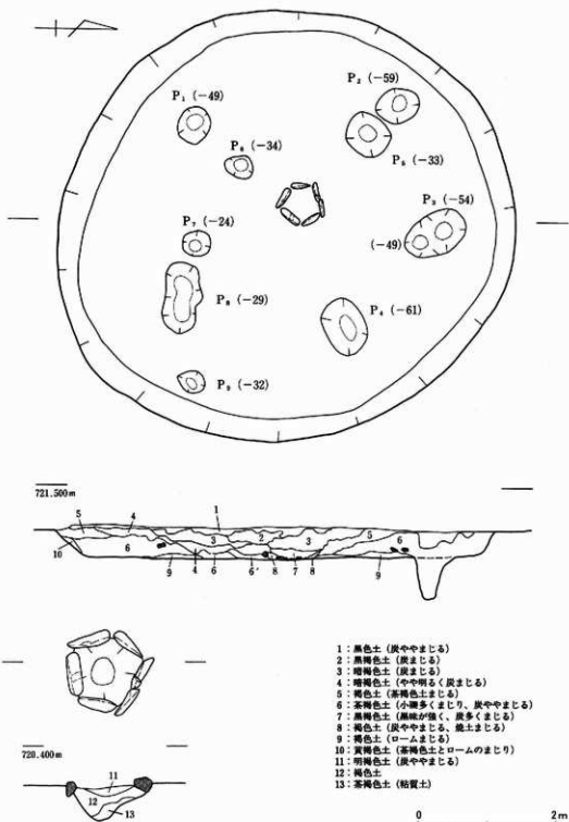
第63図 第10号住居址実測図 S = 1/60 (如: S = 1/30)
