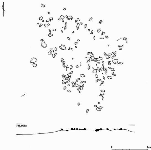
第96図 第1号集石実測図 S=1/30
