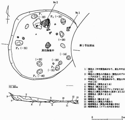
第7図 第2号住居址実測図 S = 1/60
