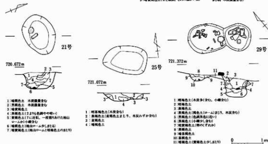
第119図 第9・10・14・20・21・25・29号土坑実測図 S=1/60
