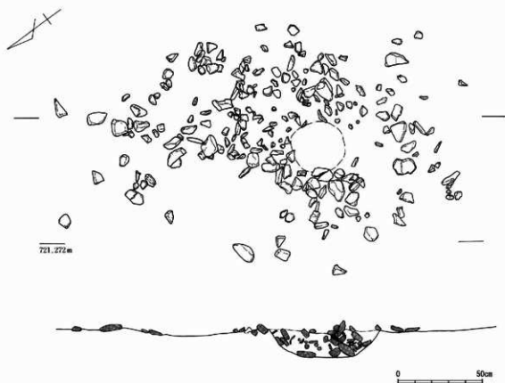
第110図 第15号集石炉実測図 S=1/20
