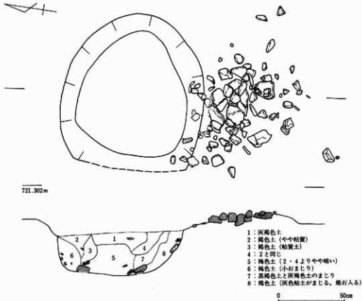
第104図 第7号集石炉実測図 S = 1/20
