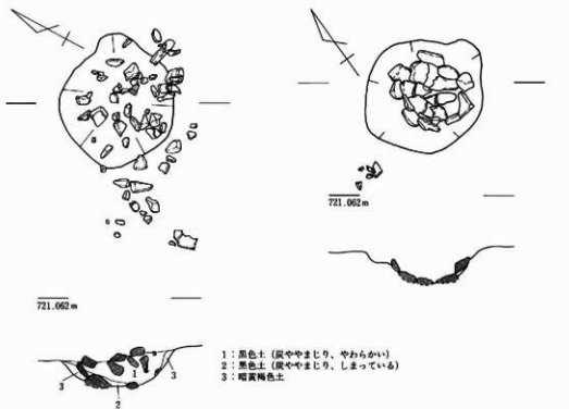
第99図 第2号集石炉実測図 S = 1/20
