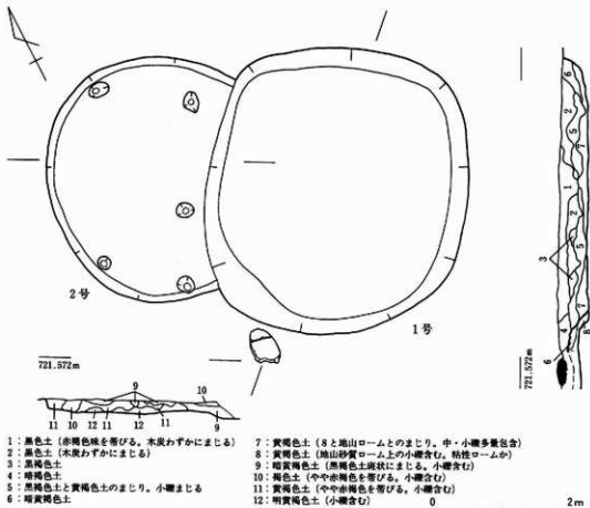
第92図 第1・2号竪穴実測図 S=1/60
