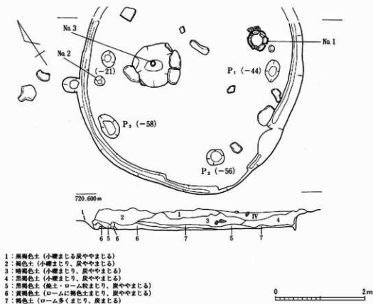
第31図 第5号住居址実測図 S=1/60
