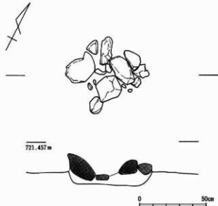
第103図 第6号集石炉実測図 S = 1/20
