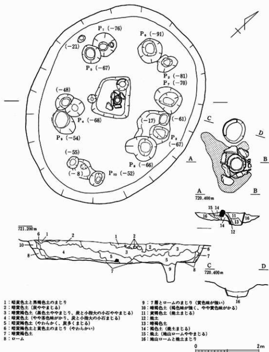
第72図 第12号住居址実測図 S=1/60 (炉: S=1/30)
