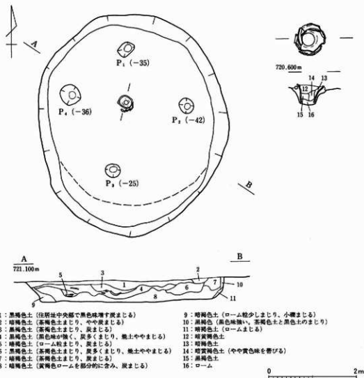
第41図 第7号住居址実測図 S = 1/60 (炉: S = 1/30)
