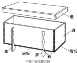
辛櫃の復原模式図
