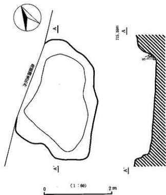
第4図 D19号土坑実測図
