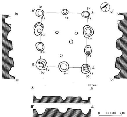
第10図 F4号掘立柱建物址実面図
