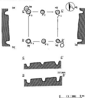
第11図 F3号掘立柱建物址実面図
