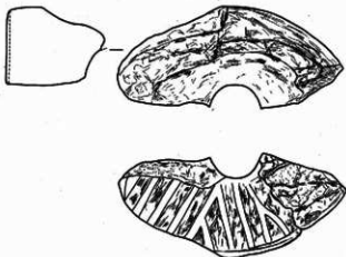
図24 石臼実測図
