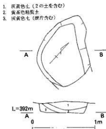
図12 土坑 208 実測図
