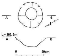
図10 土坑 206 実測図
