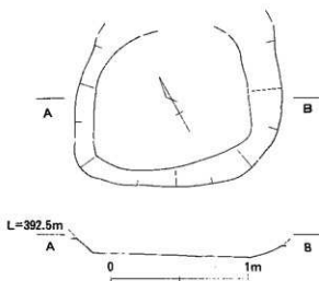
図11 土坑 207 実測図
