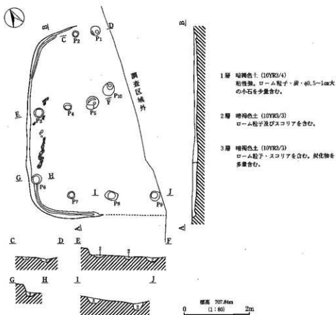
第38図 ⅢH51号住居址実測図
