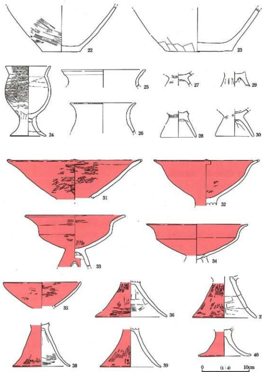
第59图 IV区埋没谷出土遗物实测图③
