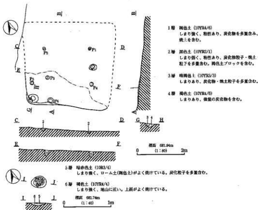
第63図 IH11号住居址実測図
