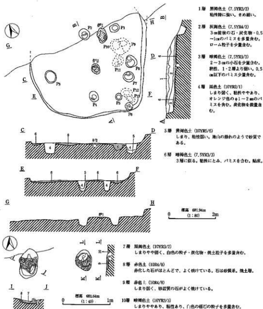
第11図 IH8号住居址実測図
