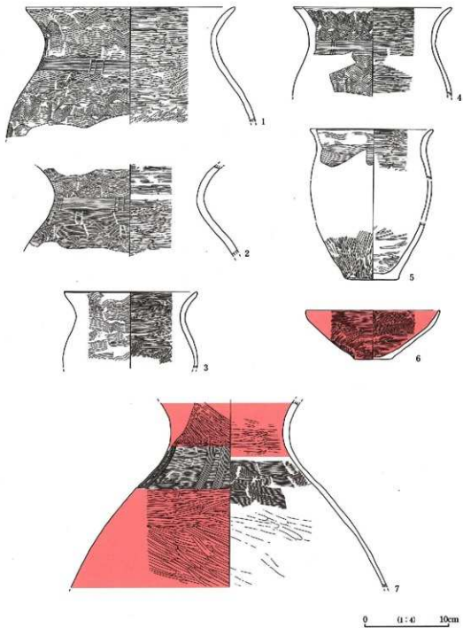
第33图 IIIH47号住居址出土物实测图②
