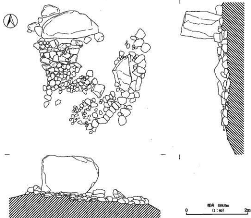
第90図 坪の内古墳石室実測図
