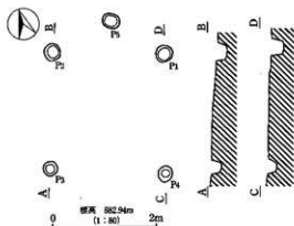
第80図 IF1号掘立柱建物址実測図
