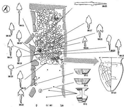
第96図 榛名平1号墳遺物出土位置図
