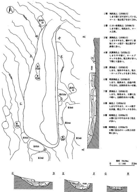
第52図 1号方形周溝基実測図
