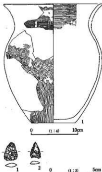
第10図 IH7号住居址出土遺物実測図
