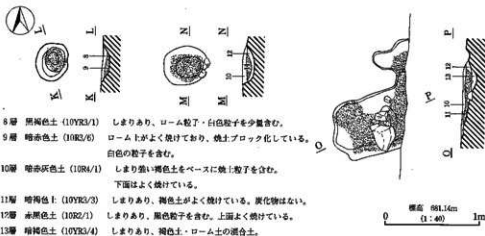
第7図 IH5号住居址実測図
