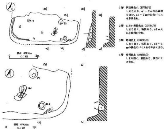
第13図 IH13号住居址及び遺物出土状況図
