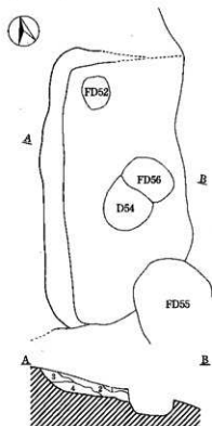
第30図 ⅢH46号住居址及び出土遺物実測図
