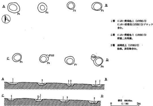
第82図 IF5号掘立柱建物址実測図
