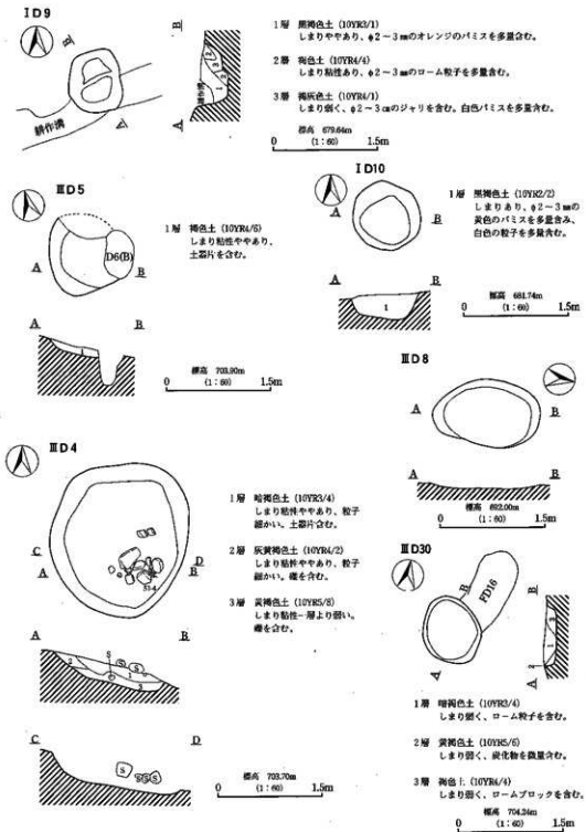
第48図 ID9-10号、ID4・5・8・30号土坑実測図
