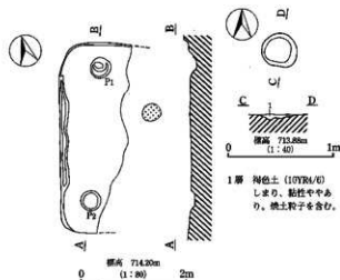
第44図 NH14号住居址実測図
