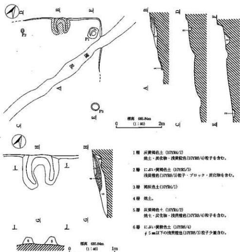
第67図 I H18号住居址実測図
