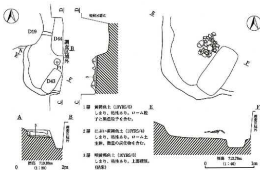
第45図 NH15号住居址実測図
