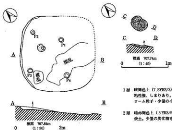
第37図 ⅢH50号住居址実測図
