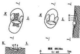
第3図 IH3号住居址実測図
