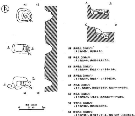
第47図 NF1号掘立柱建物址実測図
