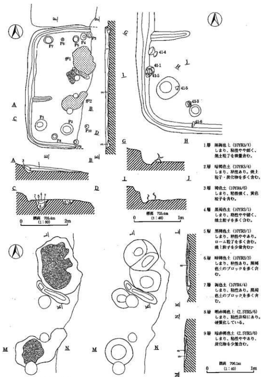
第42図 NH 8号住居址実測図
