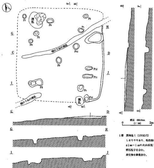
第9図 IH7号住居址実測図
