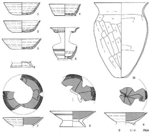
第97図 椋名平1号墳出土遺物実測図①
