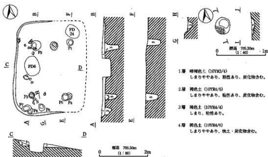
第19図 ⅢH1号住居址実測図
