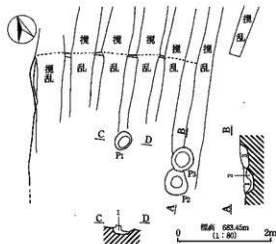
第70図 I H22号住居址実測図
