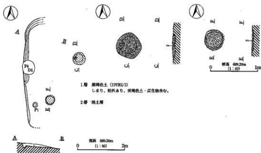
第24図 IIIH18号住居址実測図
