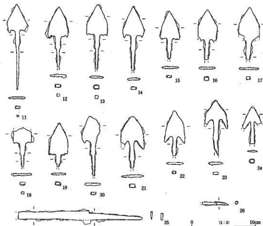
第98図 椋名平1号墳出土遺物実測図②
