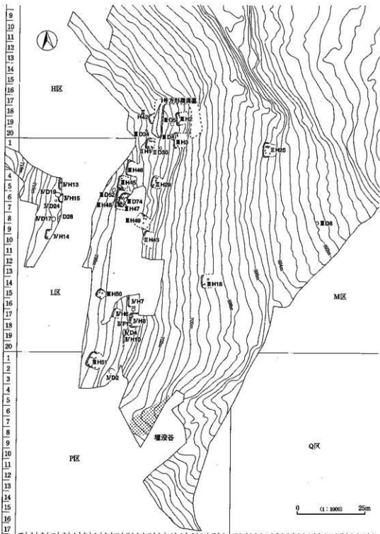
アイウエオカキクケコサシスセソタチフテト アイウエオカキクケコサシスセ 第2図 III・IV区弥生時代遺構全体図
