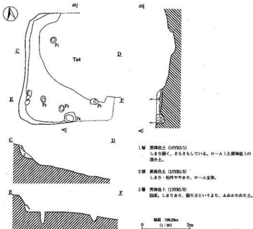
第28図 ⅢH45号住居址実測図
