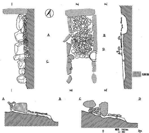
第94図 榛名平1号墳石室実測図
