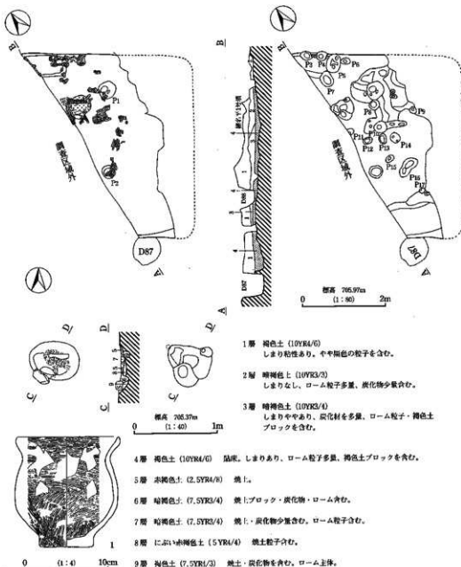
第36図 H49号住居址及び出土遺物実測図
