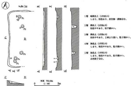
第21図 III H 2号住居址実測図
