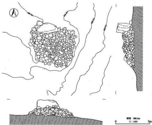
第88図 坪の内古墳検出状況図
