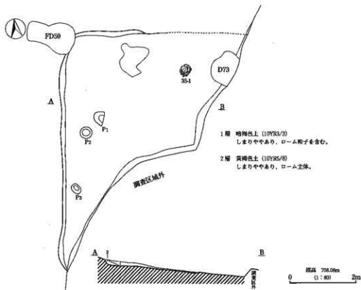
第34図 ⅢH48号住居址大測図
