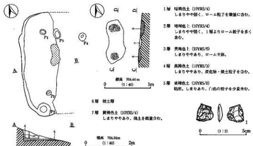
第26図 III H29号住居址及び出土遺物実測図
