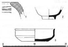
図9 SX02出土遺物実測図 (S=1/3)
