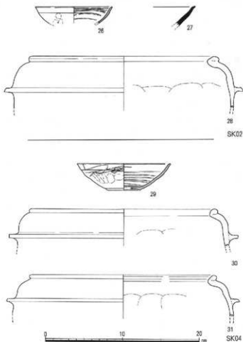
図13 第3トレンチ出土遺物実測図(S=1/3)
