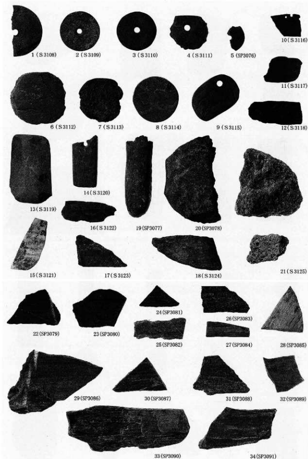
1～5 : 紡錘車、6 : 紡錘車未成品、7・8 : 円板、9 : 垂飾品、10～12 : ミニチュア石製品 13～20 : 用途不明石製品、21 : 軽石、22～28 : 石籠、29～34 : 紅崖片岩
