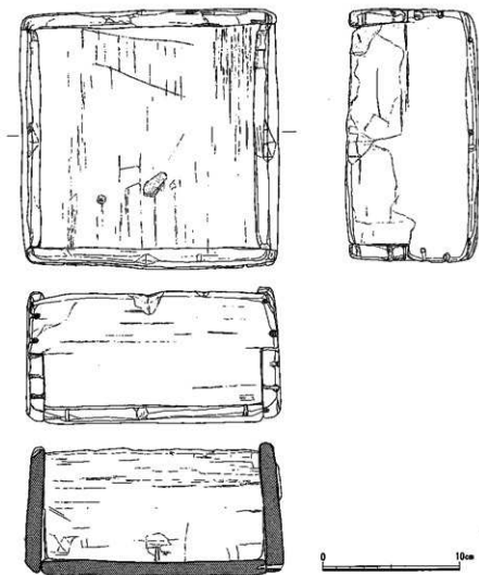
第21図 SK-2004出土木製品 (S = 1 / 3)
