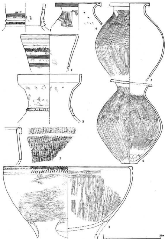
第16圖 S D-2102出土土器(1) (S = 1 / 4)
