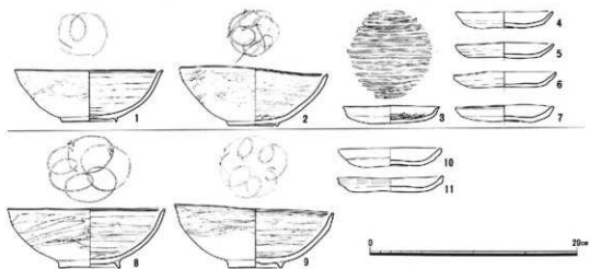
第19図 SK-2004出土土器 (S=1/4) (1～7:中層、8～11:下層)
