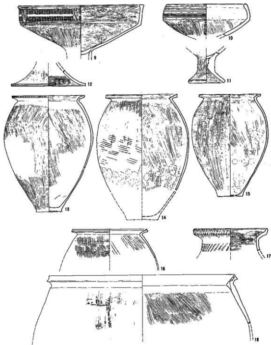
第17图 S D-2102出土土器(2) (S = 1 / 4)
