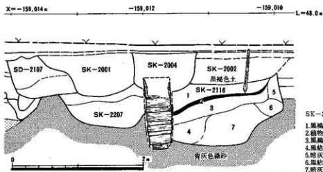
第8図 SK-2116と中世遺構西壁土層断面図 (S = 1/40)
