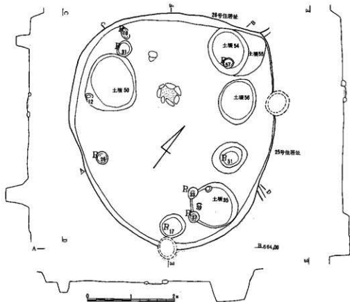
第96図 第VII地点第30号住居址実測図 (S=1/60)
