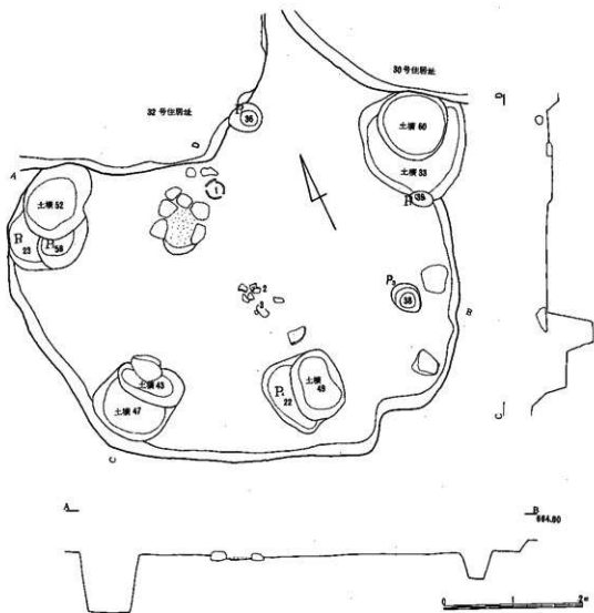
第106図 第VII地点第35号住居址実測図 (S=1/60)
