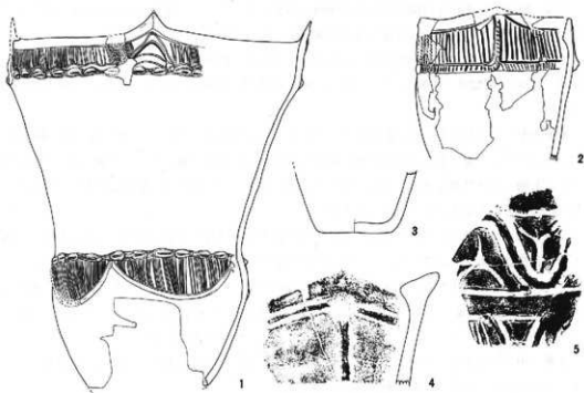
第116图 第Ⅶ地点第41号住居址床面出土土器 (1~3:1/6、4·5:1/3)
