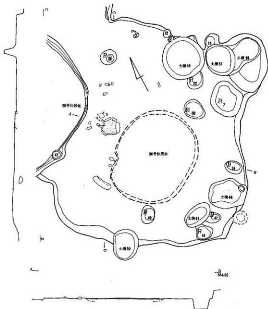
第100図 第Ⅶ地点第32号住居址実測図 (S=1/60)
