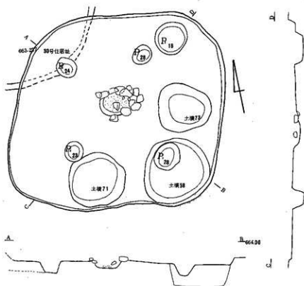
第98図 第VII地点第31号住居址実測図 (S=1/60)
