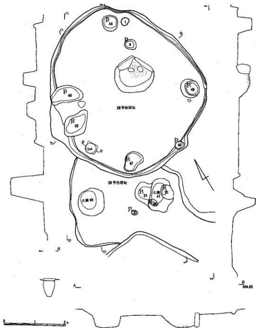
第91图 第七地点第28号·29号住居址实测图 (S=1/60)
