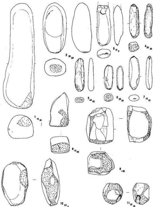
第141图 敲打器 (a·b类) 实测图 (1/3 1~7为a类、8~11为b类)
