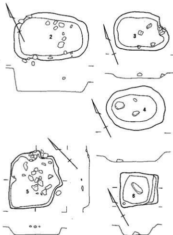
第131図 第七地点歴史時代土坑実測図 (S=1/60)
