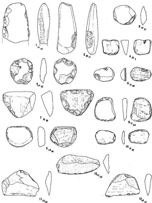
第142図 敲打器(c類) 特殊敲打器、横刃形石器実測図 (1/3 1・2は敲打器c、3~10は特殊敲打器、11~13は横刃形石器)
