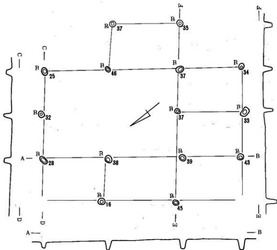
第128図 第VII地点第7号建物址実測図 (S=1/80)
