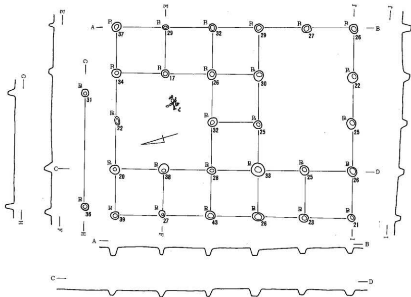
第122图 第七地点第1号建筑物实测图 (S=1/80)
