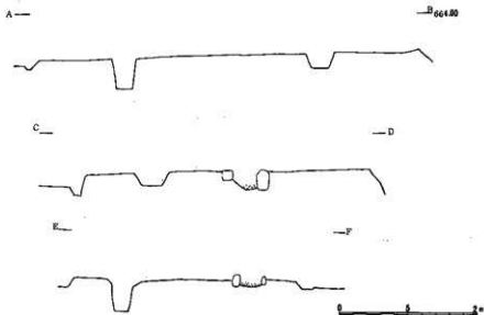
第88图 第VII地点第26号·27号住居址实测图 (S=1/60)
