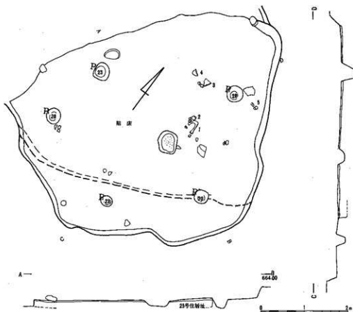
第81図 第VII地点第24号住居址実測図 (S=1/60、5は石錘4点)
