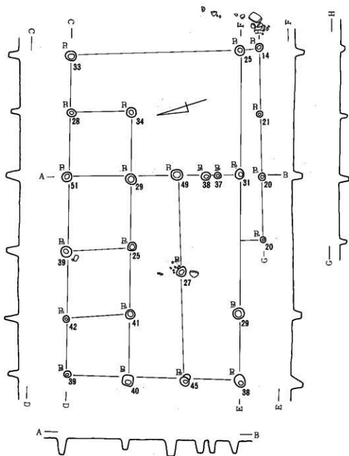
第125图 第七地点第4号建物址实测图 (S=1/80)
