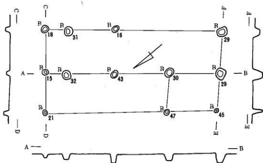
第127図 第Ⅶ地点第6号建物址実測図 (S=1/80)
