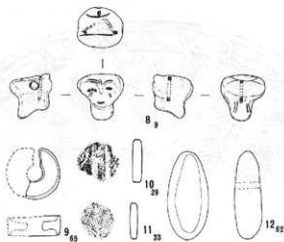
第121図 第七地点土壌出土土製品及び石製品（1/3、小数字は出土土壌番号）
