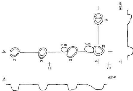
第2号掘立柱建物跡
