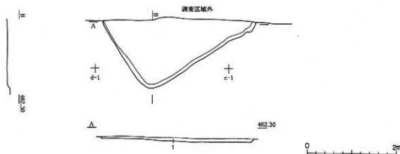
第2号竪穴住居跡
