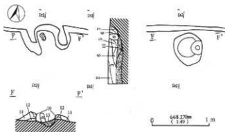
第35図 H13号住居址・遺物実測図
