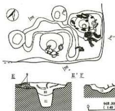
第20図 H7号住居址実測図(2)
