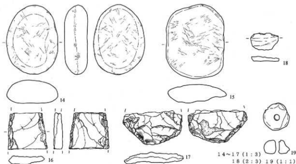
第43図 M1号溝状遺構遺物実測図(2)
