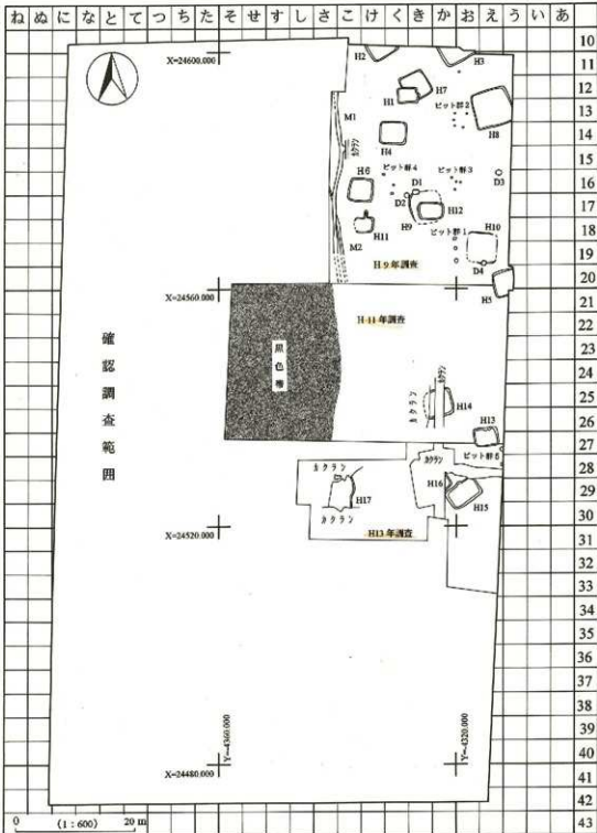
第5図 中遺跡跡Ⅱ遺構配置図 (1:600)
