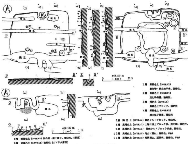
第13図 H4号住居址実測図
