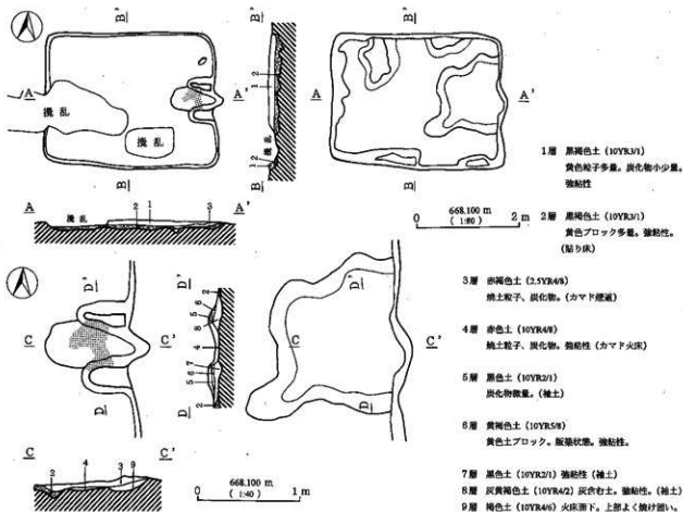
第6図 H1号住居址実測図
