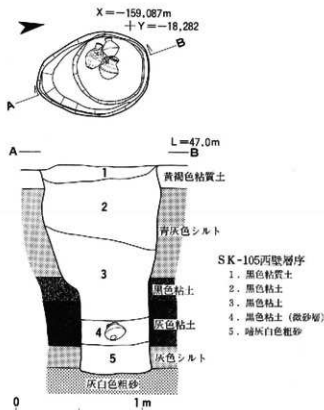
第7図 SK-105遺構平面及び断面図 (S=1/6)
