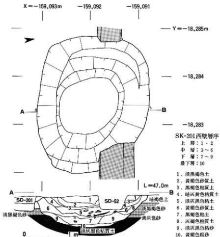
第4図 SK-201遺構平面図及び断面図 (S=1/6)
