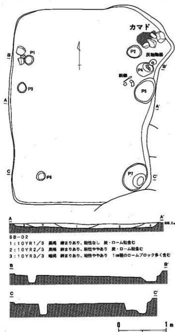
第5図 SB-02実測図
