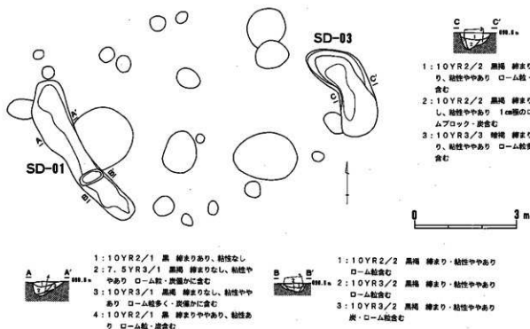
第8図 SD-01・03実測図
