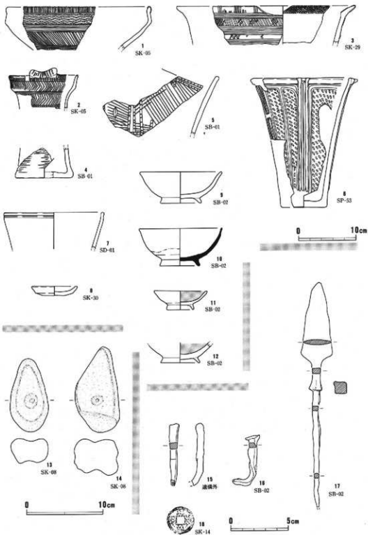
第9圖 出土遺物実測図
