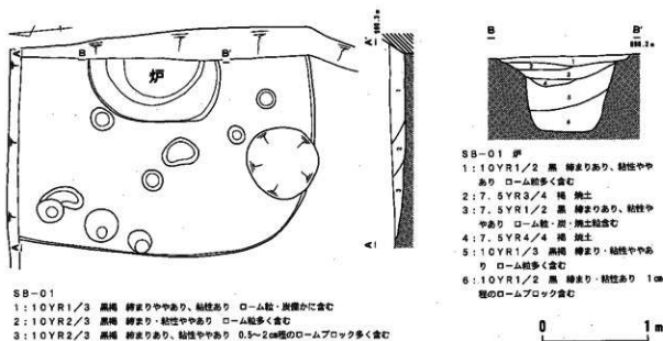
第3図 SB-01実測図
