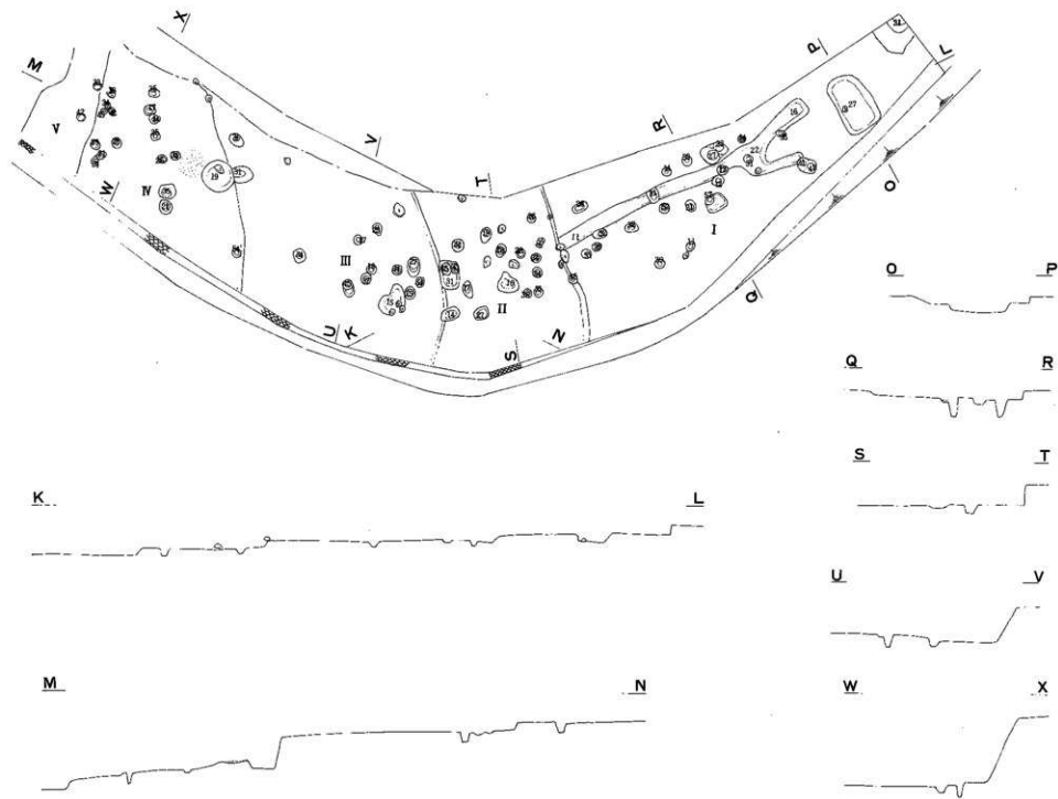
第7図 遺構実測図 (S = 1:120) (水系レベル±620.00m)
