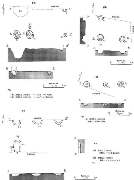
第47図 F5・F7・F8・F9号掘立柱建物跡実測図
