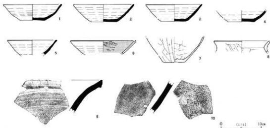
第22図 H12号住居址実測図および出土遺物実測図
