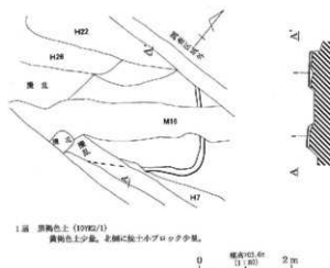
第16図 H8号住居址実測図
