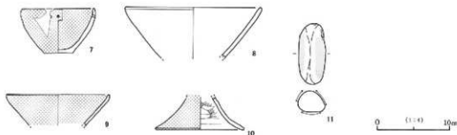
第12図 H5号住居址出土遺物実測図
