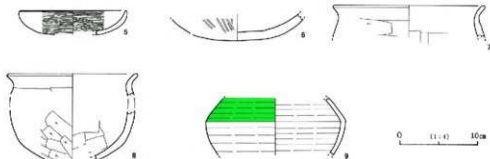
第32図 H17住居出土遺物実測図
