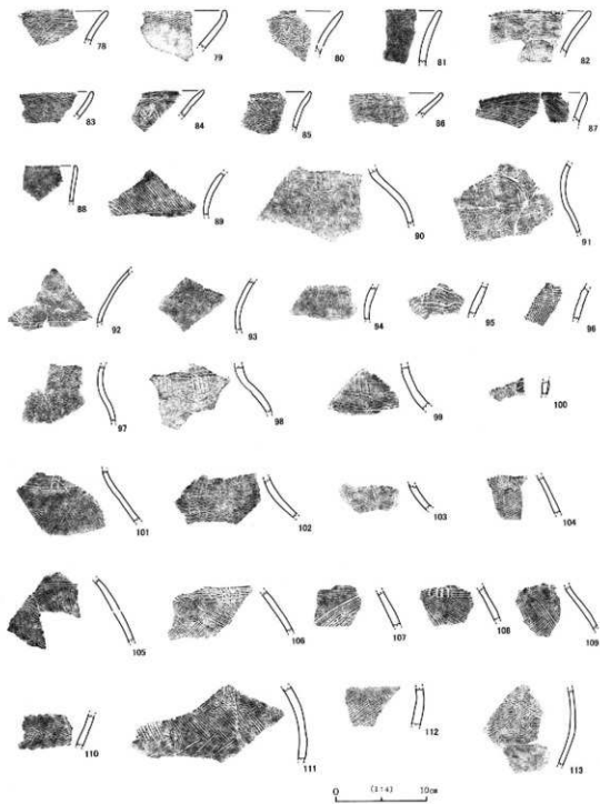
第59图 M1·M2号洞状遗物出土器物实测图
