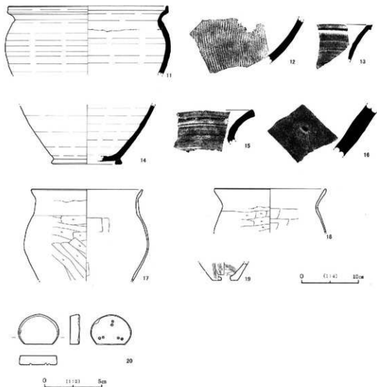
第30図 H16号住居址出土遺物実測図
