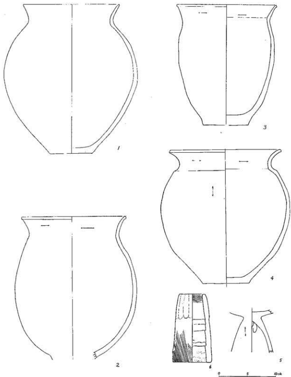
第17图 1号祭祀遗址出土土器实测图
