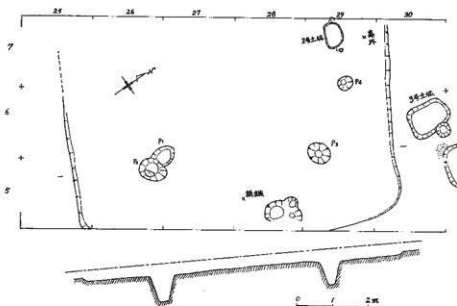
第5图 H-2号住居址平面图
