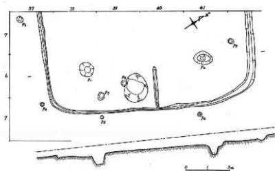
第6图 H-3号住居址平面图
