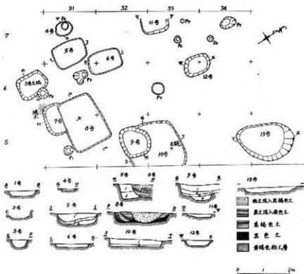
第7图 土着群平面图
