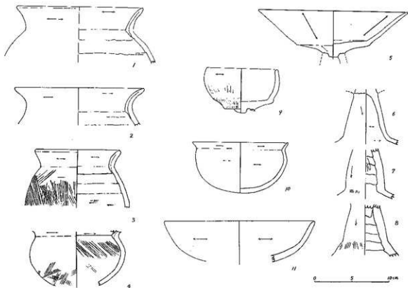
第16図 H-3号住居址出土土器実測図
