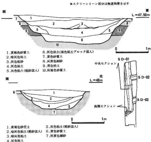
第12図 SD-01土層断面図
