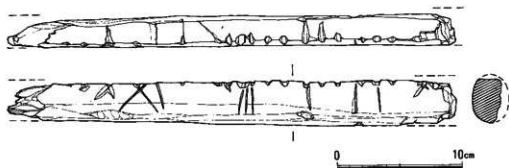
第19図 SE-03出土「棒はかり」状木製品(S=1/3)
