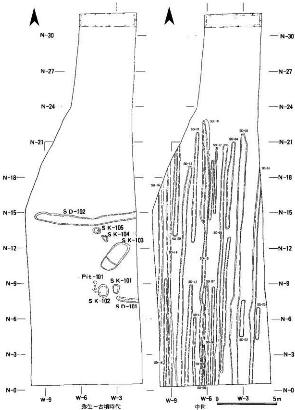
第6図 第2次調査遺構平面図
