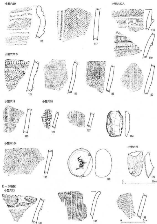
第113图 小整穴69·20A·20B·18·19·75·104·13出土石器拓影、石器实测图 116~123·125~127·130~133 (1:2) 124·128·129 (1:3)
