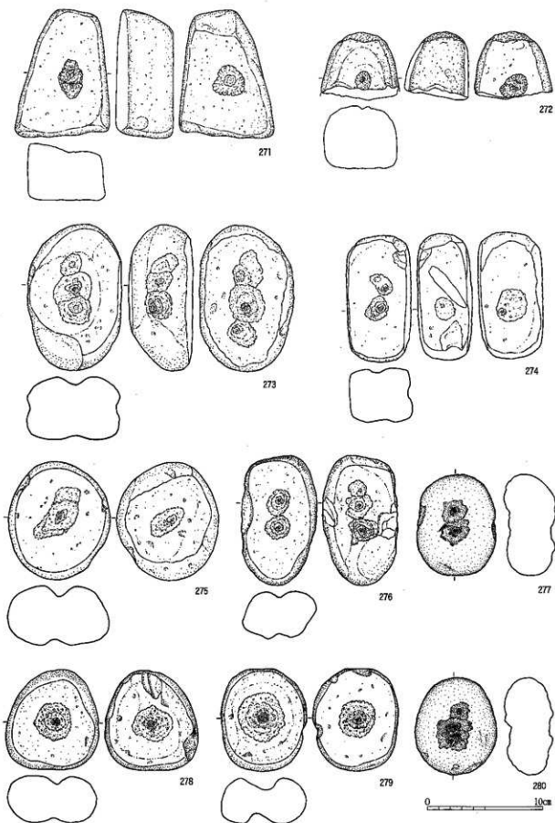
第135图 遗孀外出石器实测图 (1 : 3)
