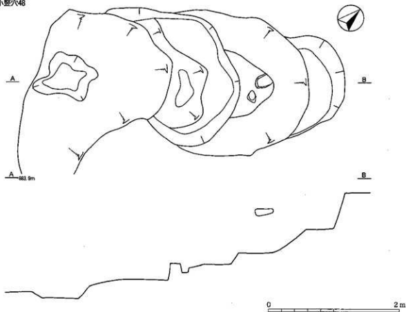
第142圖 小豎穴47・48実測圖(1:40)
