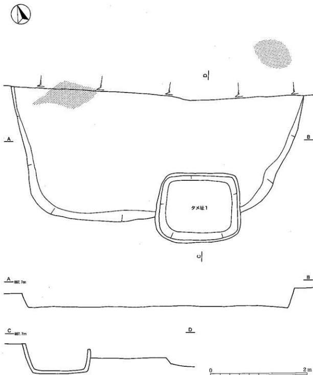
第140図 第4号竪穴住居址・タメ址実測図 (1 : 40)
