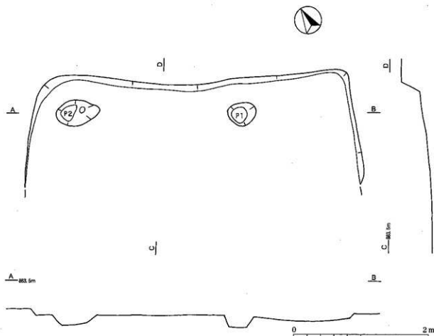
第141図 第20号竪穴住居址実測図（1：40）
