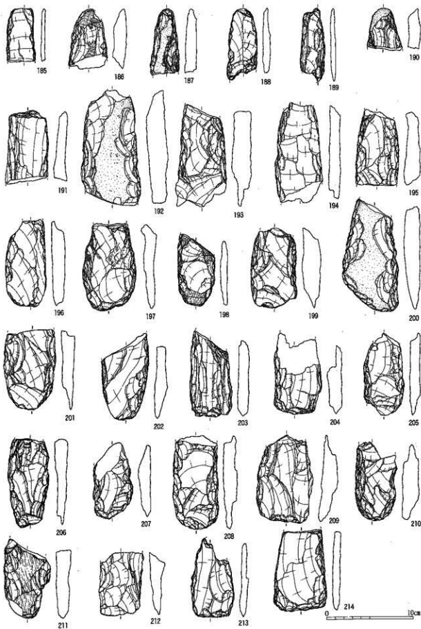
第132图 遼博外出石器类图(1:3)
