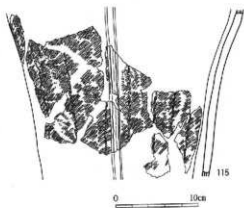
第112图 小墅穴74·106·17·14出土石器·石器实测图、石器拓影 105·106·113 (1:3) 107~112 (1:2) 114·115 (1:4)
