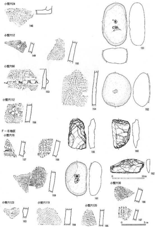
第115图 小箭头24·12·66·112·78·119·120·123·6·30出土石器拓影、石核实例图 148~150·153·154·156·157~159·163~167 (1:2) 151·152·155·160~162 (1:3)
