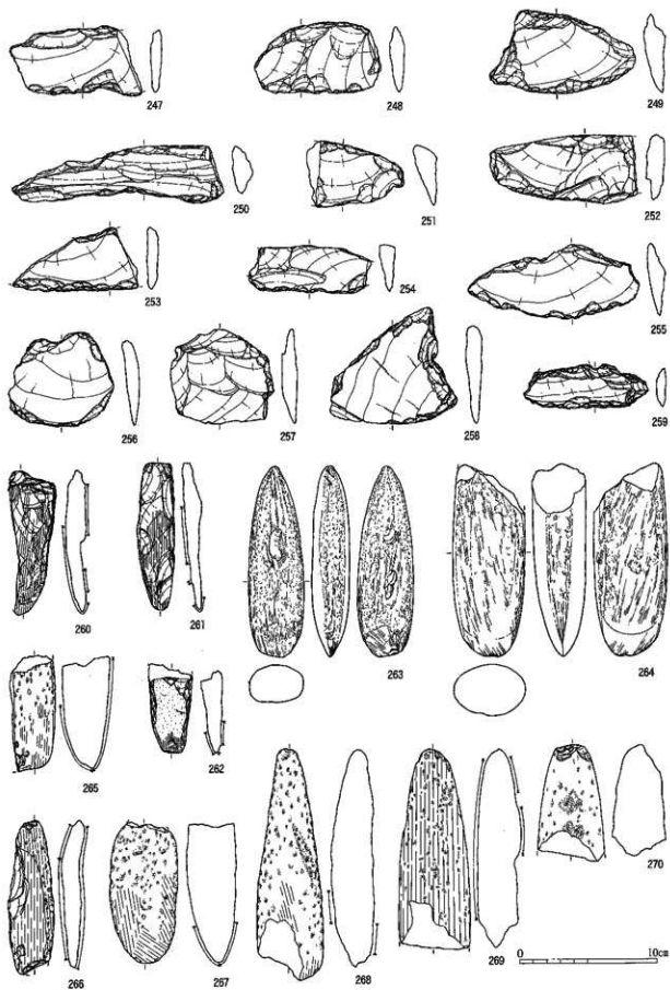
第134图 遺構外出石器実測図 (1:3)
