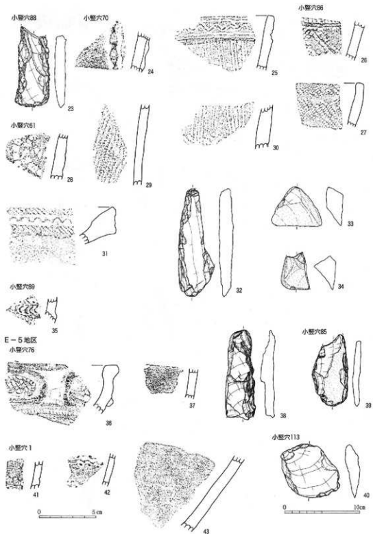
第107图 小整穴88·70·86·61·89·85·76·113·1出土土器拓影、石器实图 23·32~34·38~40(1:3) 24~31·35~37·41~43(1:2)
