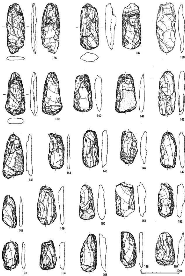
第130圖 遺構外石器等實測圖 (1:3)
