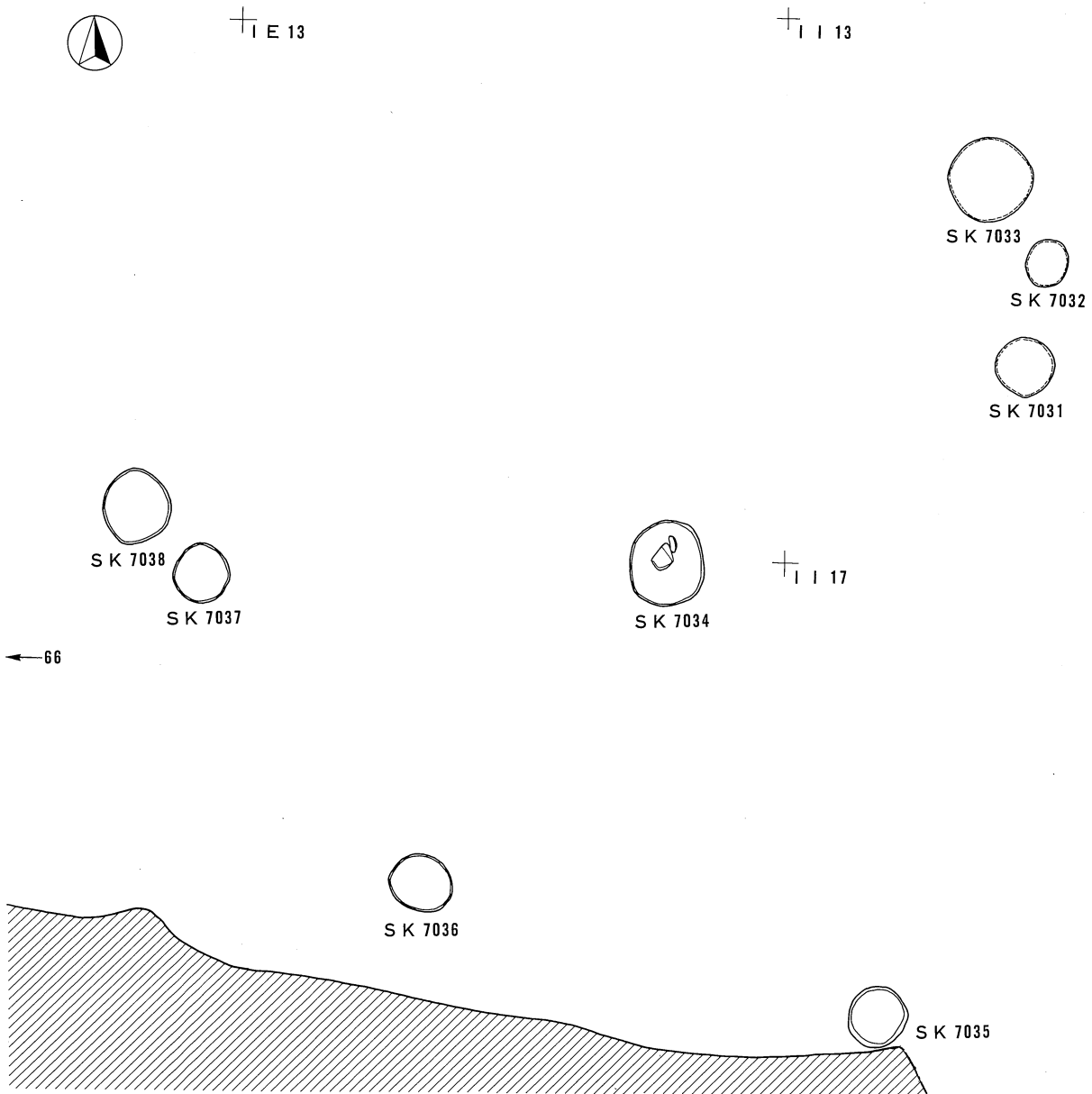
割付图 70
