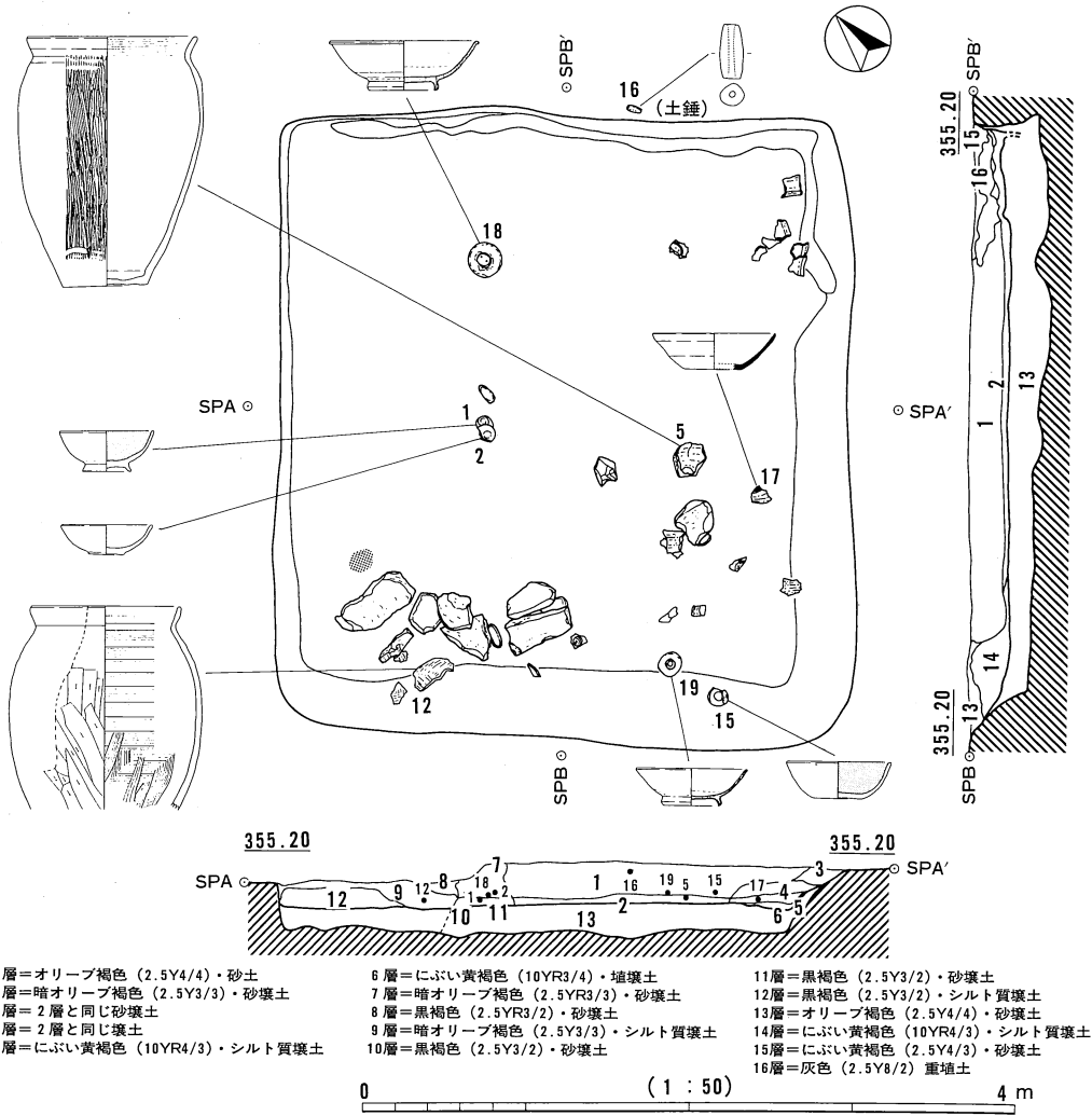
SB7053個別図
