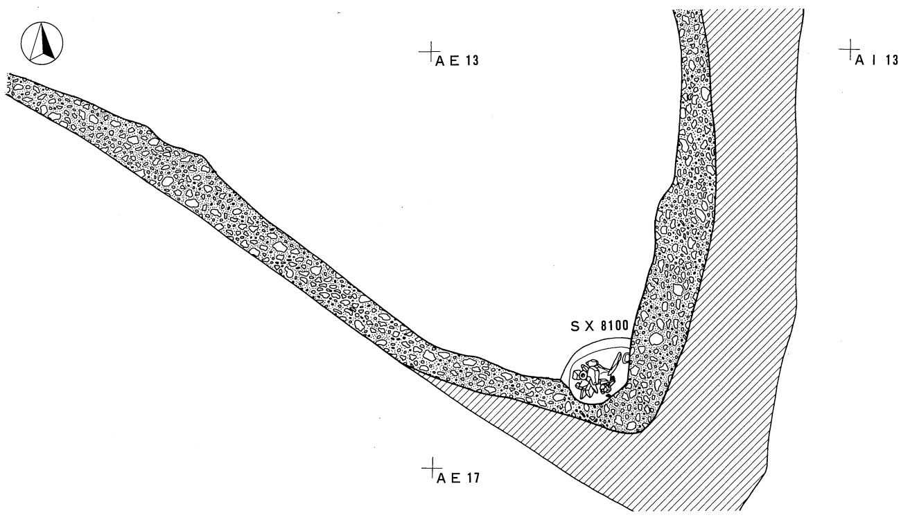
割付図 28
