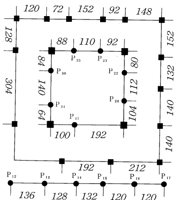
挿図9 岡田町遺跡D区第3005号住居址柱構造変遷模式図 (cm)
