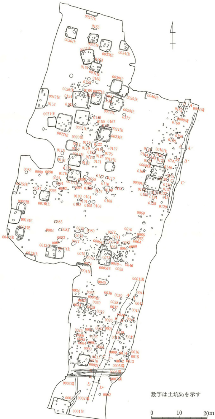
挿図6 岡田町遺跡A区遺構配置図
