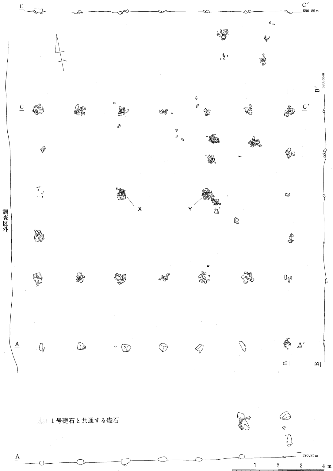
第10図 礎石(3)
