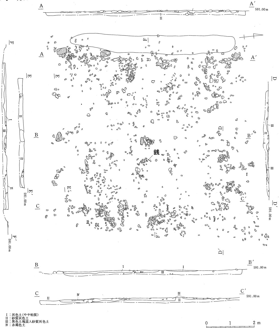
第8図 礎石(1)
