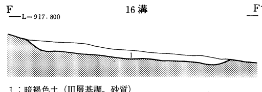
第391図 溝址断面図
