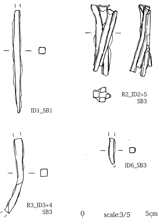
第7図 金属製遺物実測図
