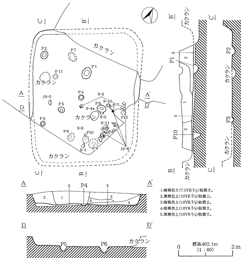
第8図 Y2号住居址実測図
