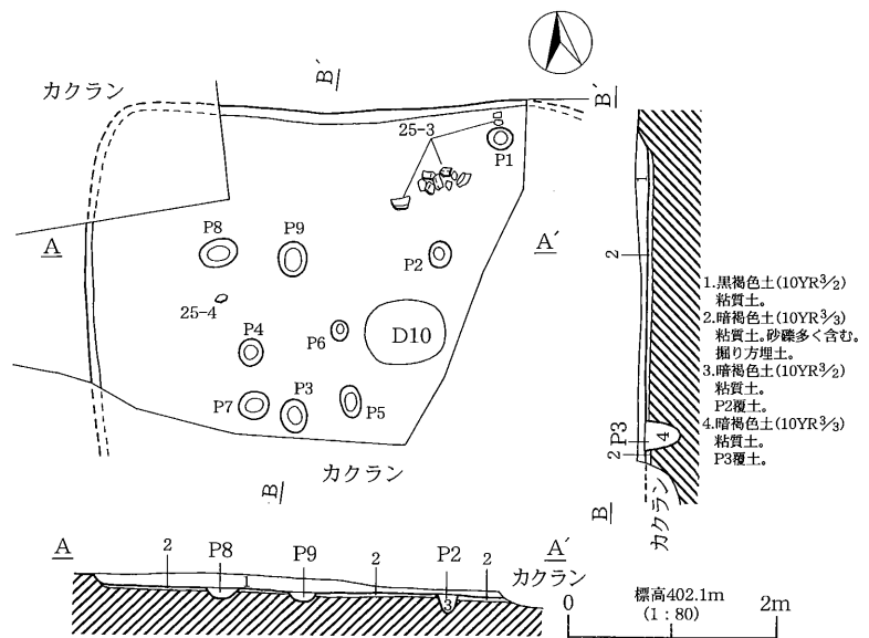
第24図 Y6号住居址実測図
