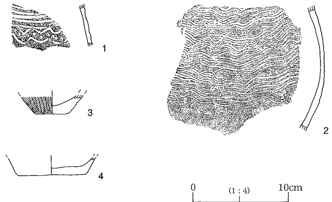
第27図 Y7号住居址 出土土器実測図
