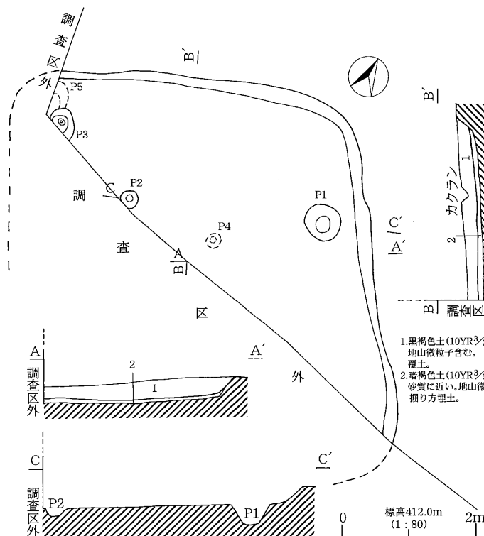
第15図 H1号住居址実測図
