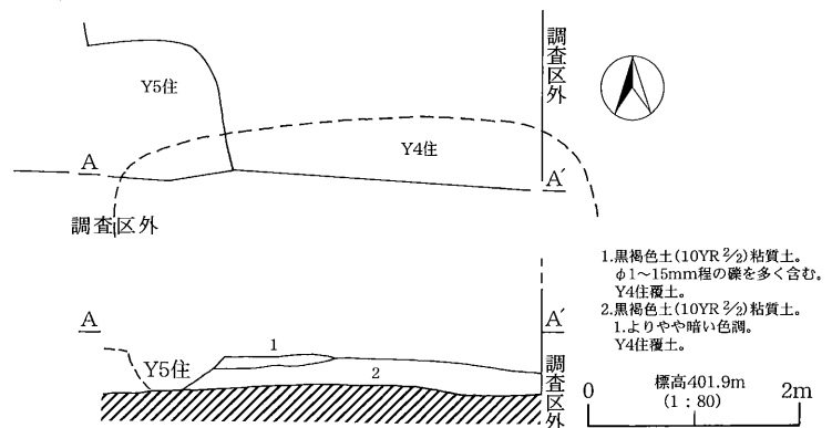
第13図 Y4号住居址実測図
