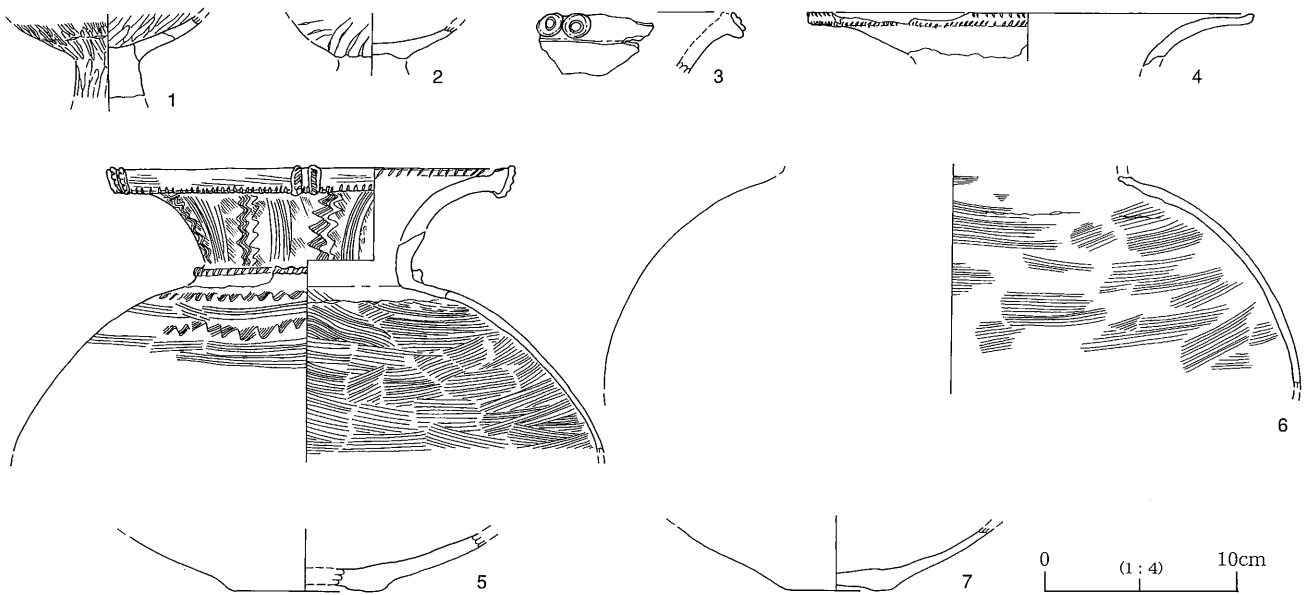
第12図 Y3号住居址出土土器実測図
