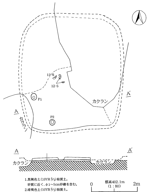
第11図 Y3号住居址実測図
