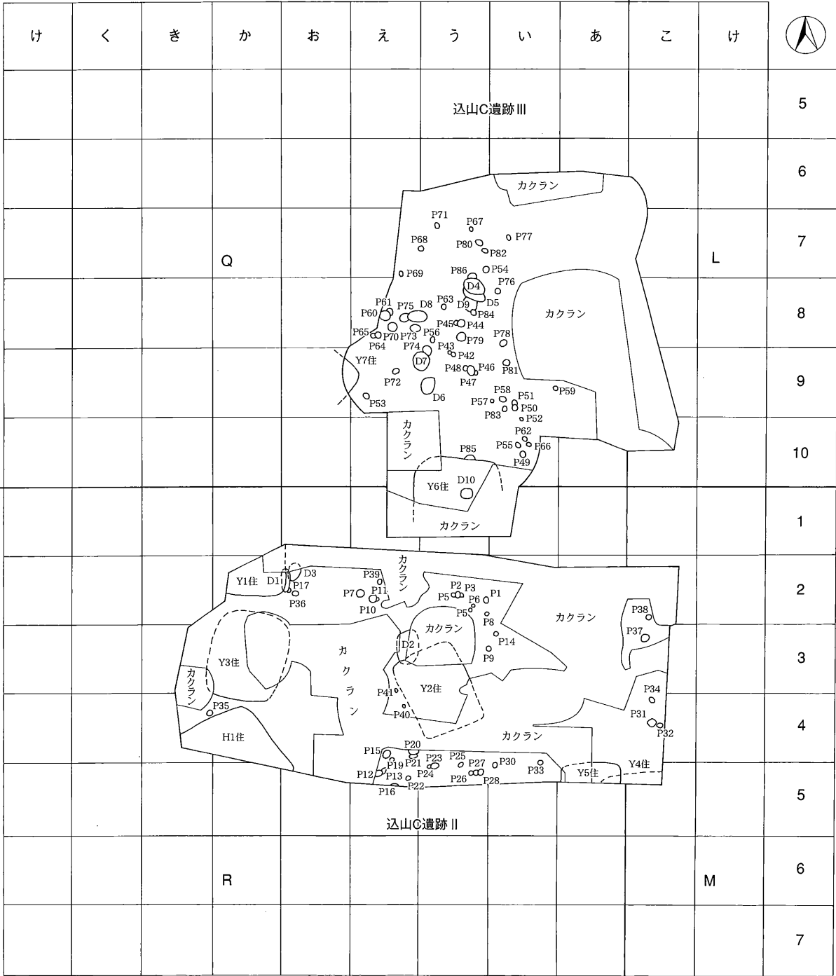
第23図 込山C遺跡Ⅲ 遺構配置図 (1 : 300)
