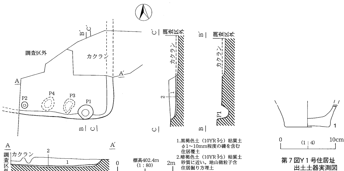
第6図 Y1号住居址実測図
