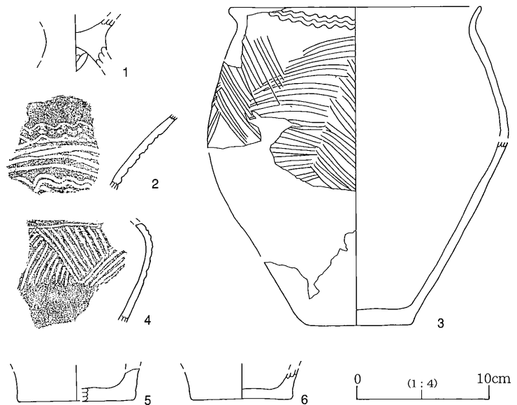
第25図 Y6号住居址出土土器実測図
