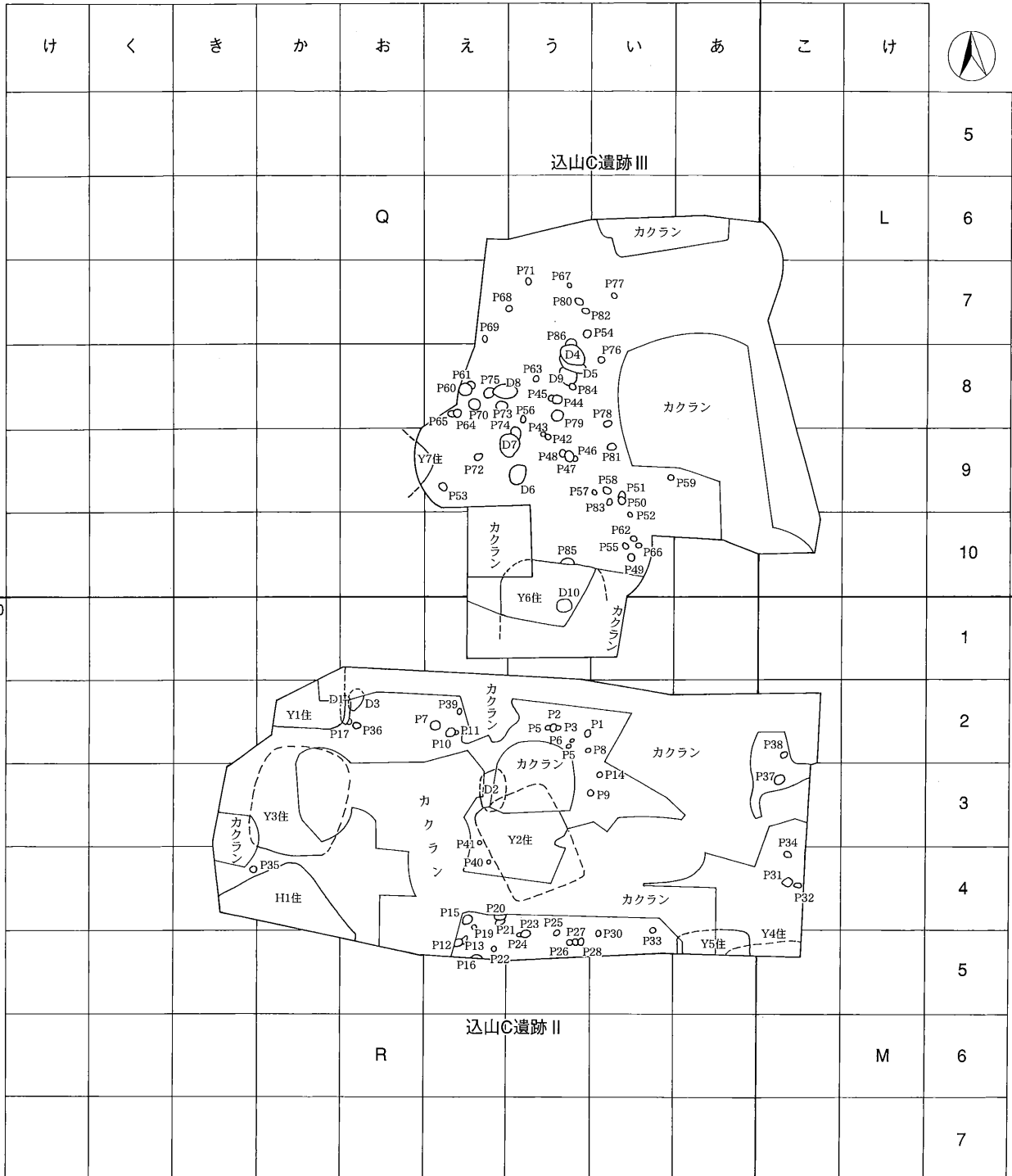
第5図 込山C遺跡II 遺構配置図 (1:300)
