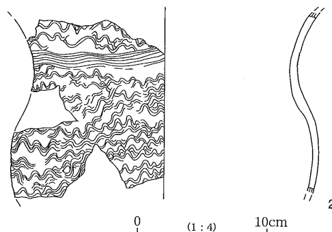
第29図 D 6号土坑址 出土土器実測図
