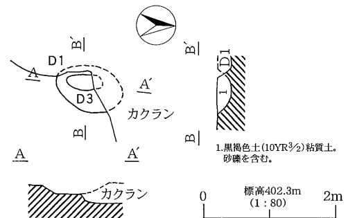
第17図 D1~D3号土坑址実測図
