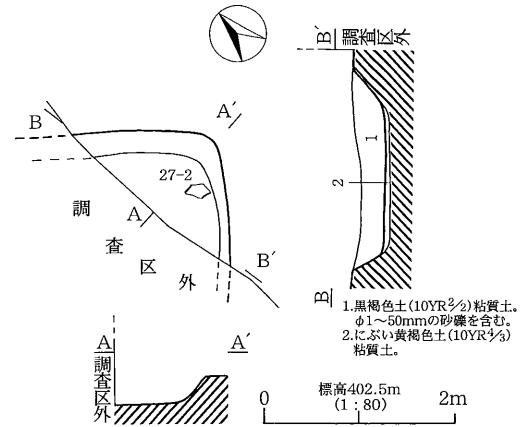
第26図 Y7号住居址実測図
