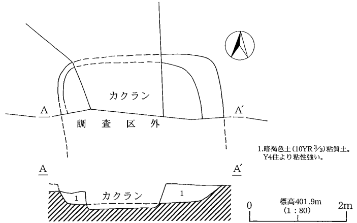
第14図 Y5号住居址実測図
