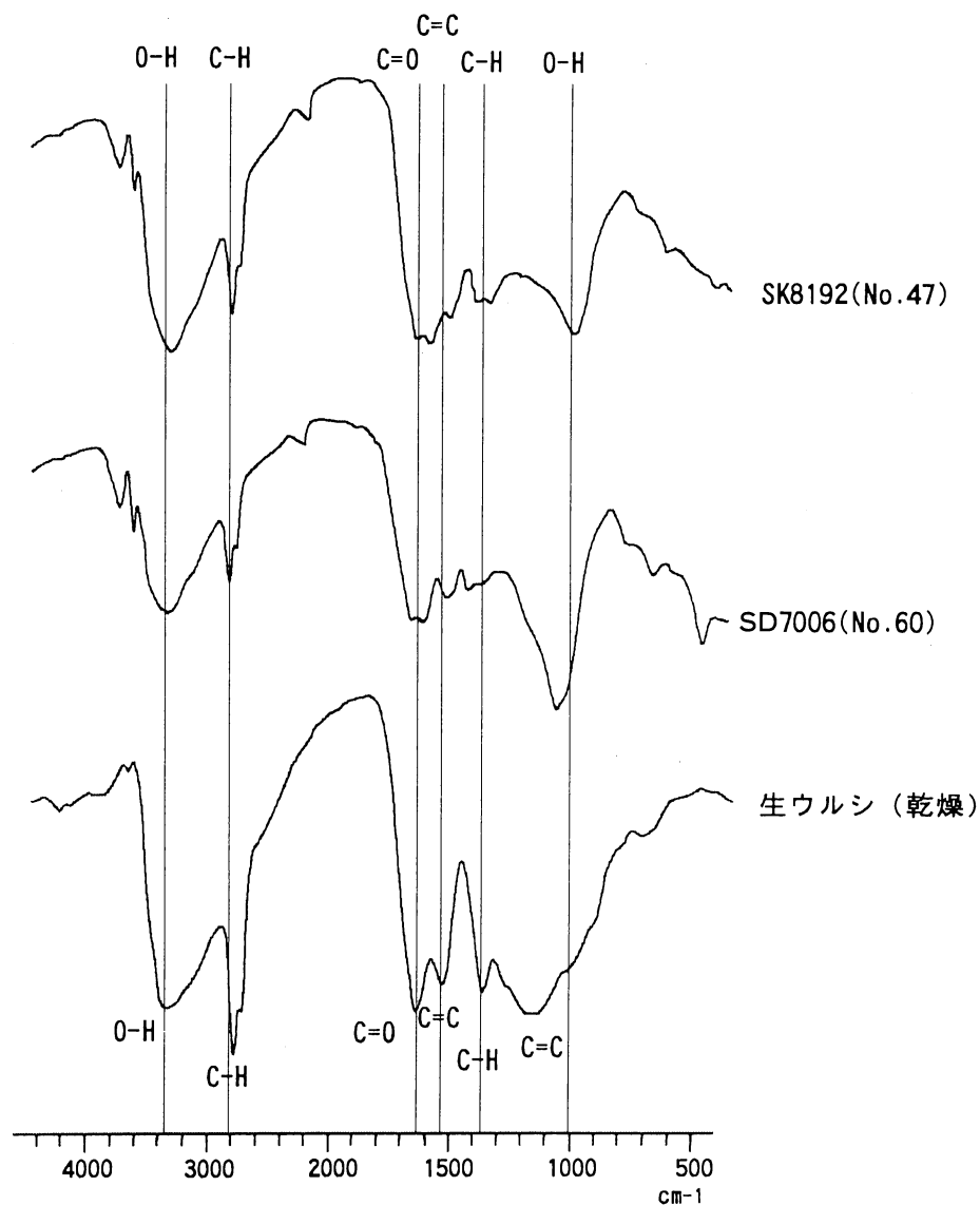
第86図 ウルシ状付着物と生ウルシ (乾燥) の赤外吸収スペクトル
