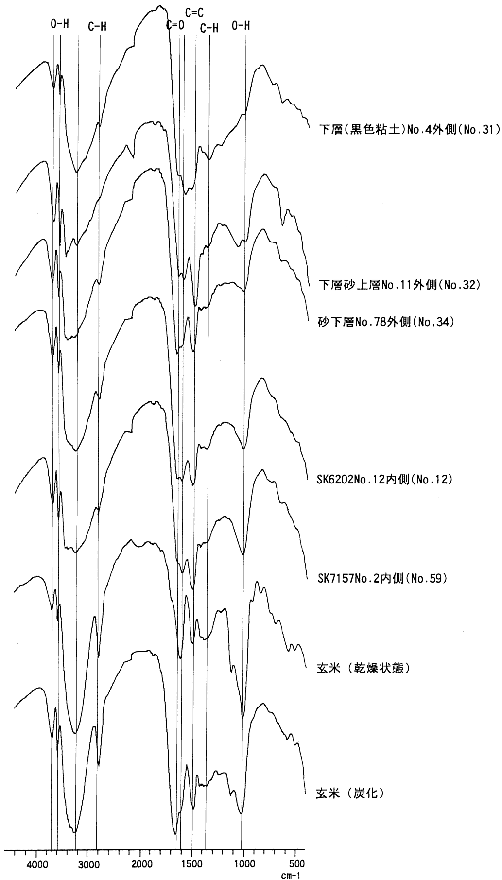
第87図 オコゲ状附着物と対照試料の赤外吸収スペクトル
