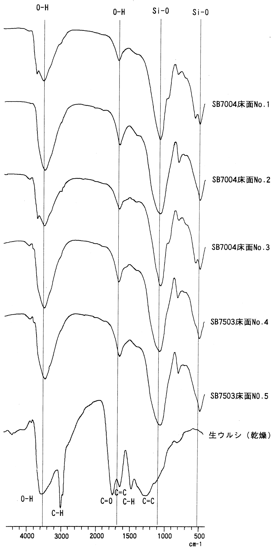
第85図 黒色物質と生ウルシ (乾燥) の赤外吸収スペクトル
