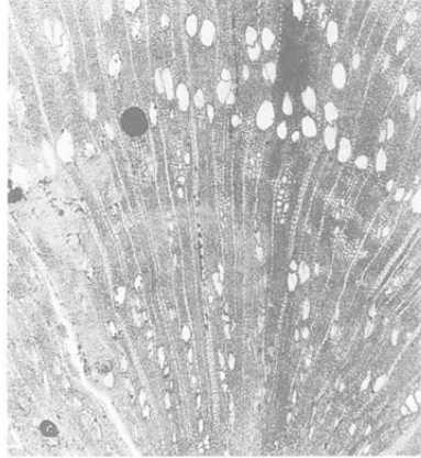
49 a ハギ属 bar:1mm NAG 21327
