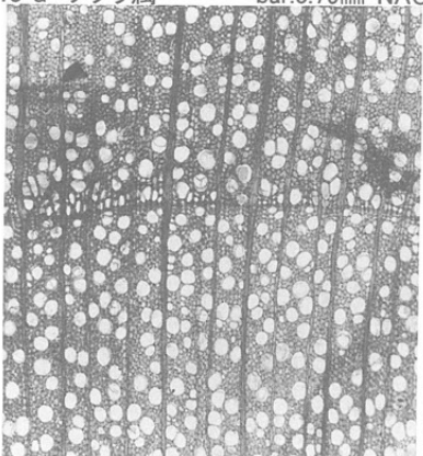
44 a ナシ亜科 bar:0.75mm NAG 20589
