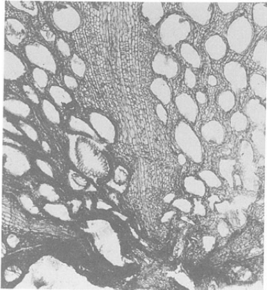
24 a クヌギ節根材 bar:1mm NAG 22156
