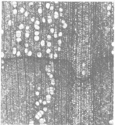
15 a ハノキ属ハノキ節 bar:0.75mm NAG 20485
