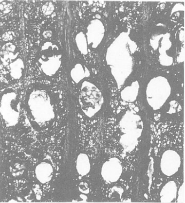
63 a ツルウメモドキ
