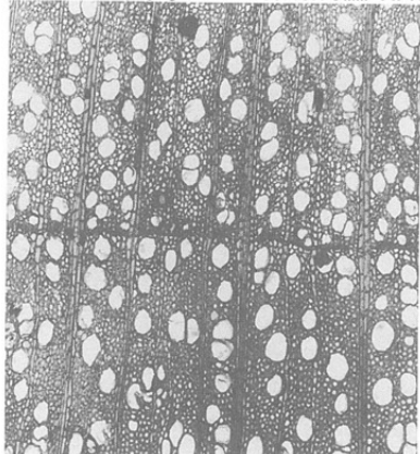
43 a サクラ属 bar:0.75mm NAG 21870
