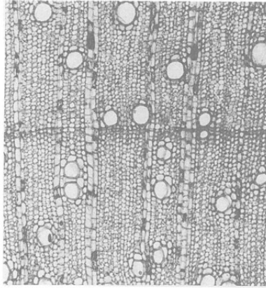
61 a アワブキ
