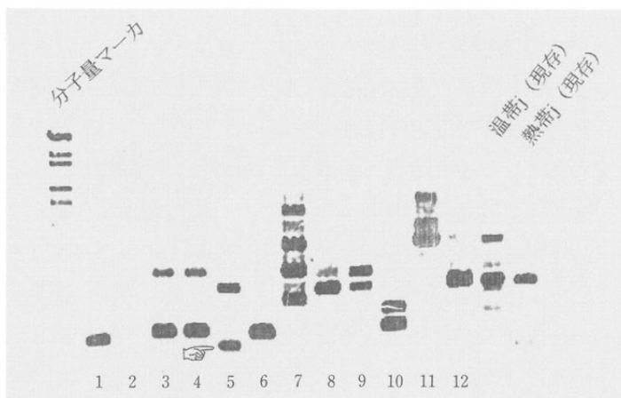
写真1 川田条里遺跡出土の稲サンプルのDNA電気泳動写真
