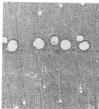
79 a トネリコ属
