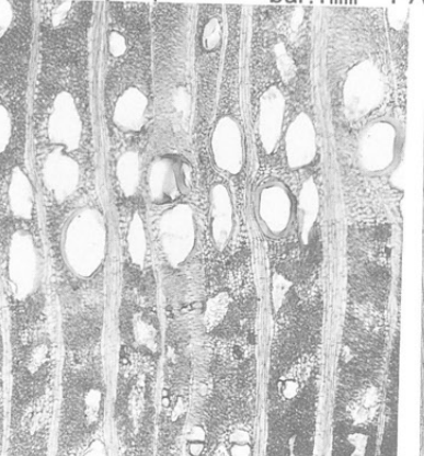
48 a サイカチ bar:1mm NAG 22567
