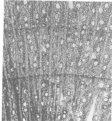
78 a サワフタギ類
