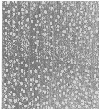
85 a ガマズミ属 bar:1mm PAL 682
