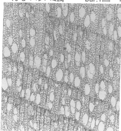
20 a アサダ bar:0.75mm
