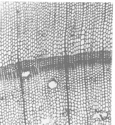
4 a アカマツ bar:0.75mm NAG 570
