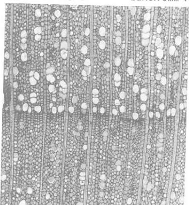
32 a モクレン属
