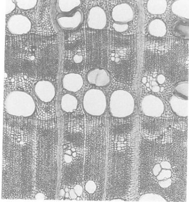
45 a フジキ bar:1mm PAL 839
