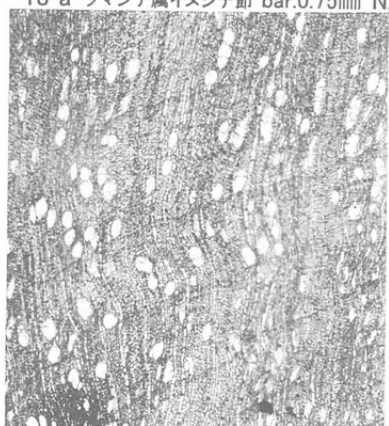
19 a ハシバミ属 bar:1mm
