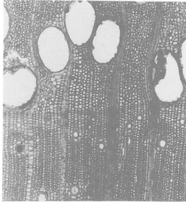
65 a ケンパンシ属 bar:0.75mm NAG 20070
