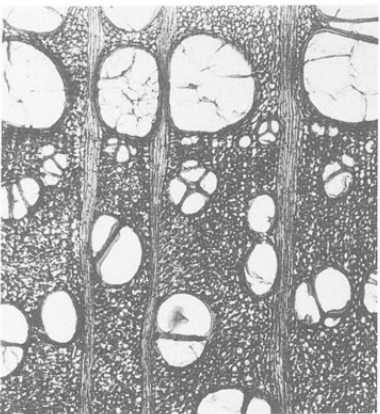
88a クワ bar:0.64mm PAL805
