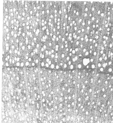
40 a カマツカ bar:1mm NAG 20541
