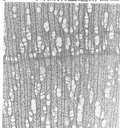
17 a クマシデ属クマシデ節 bar:1mm
