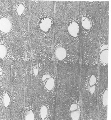
47 a ユクノキ bar:1mm PAL 951
