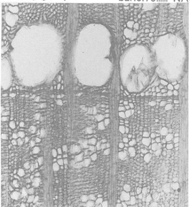
75 a ハリギリ bar:0.75mm NAG 20392
