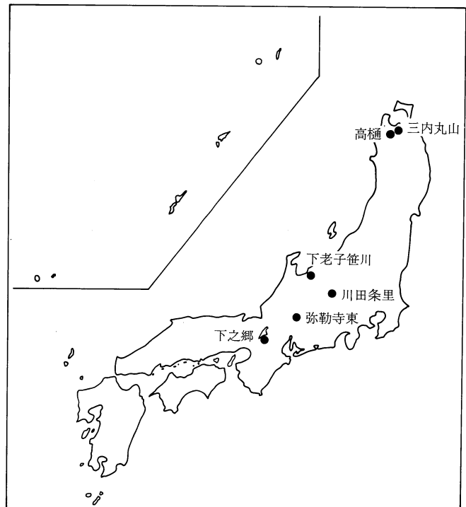
図1 DNA分析 試料採取遺跡
