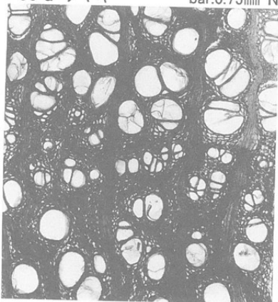
31 a ヤマゲワ
