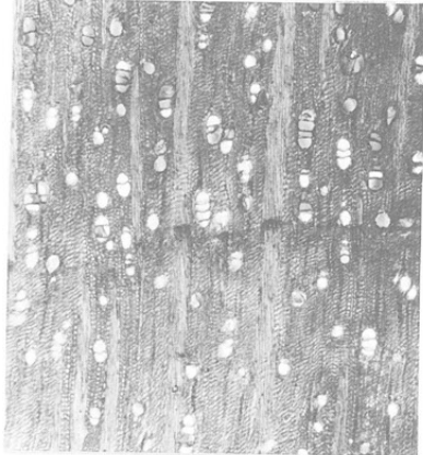
59 a カエデ属根材
