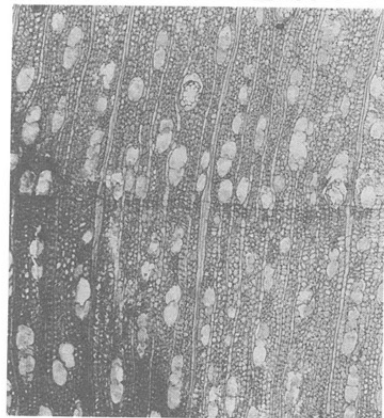
77 a エゴノキ属
