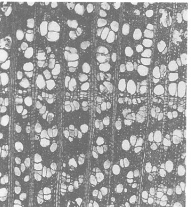
84 a ニワトコ
