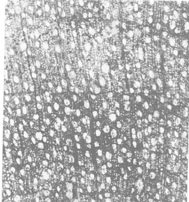
70 a キブシ根材
