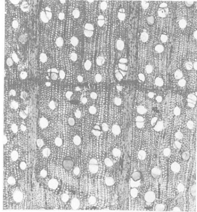
57 a チドリノキ
