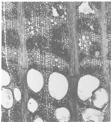
86a エノキ属 bar:0.64mm NAG20496
