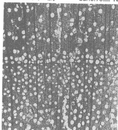
80 a イボタキ属
