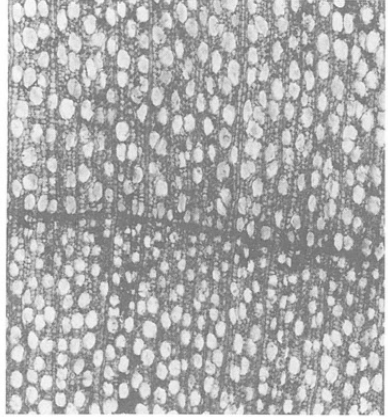
14 a ヤナギ属 bar:0.75mm NAG 20430
