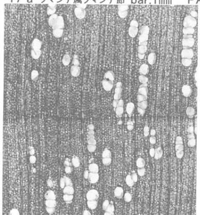
18 a クマシデ属イヌシデ節 bar:0.75mm
