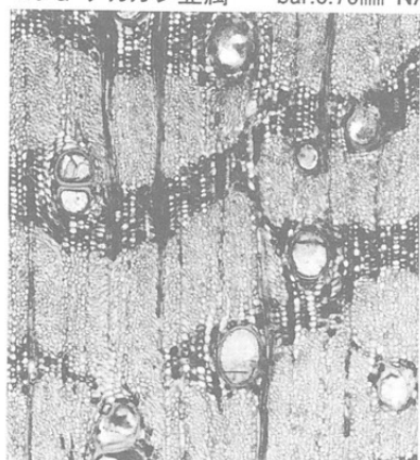
27 a ムクノキ
