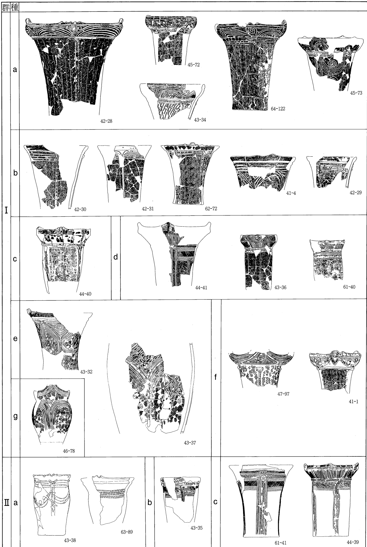
第97図 縄文時代中期初頭の土器群
