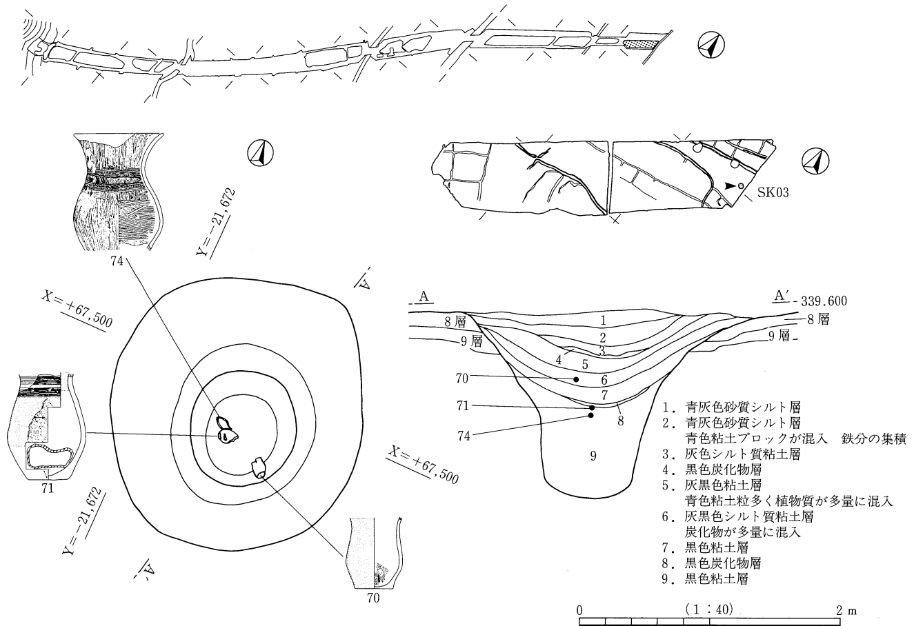
第164図 E2地区第4A調査面SK03平面・断面図
