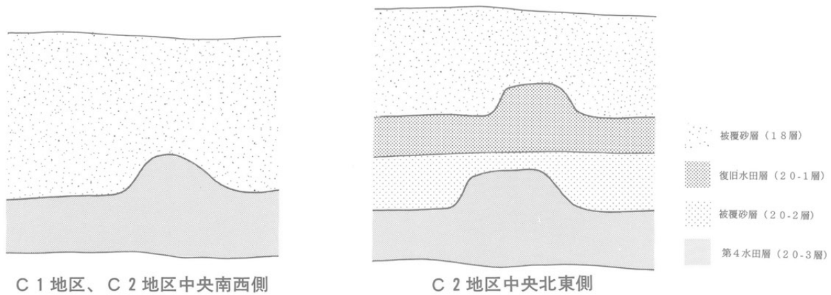
第92図 C地区第4水田被覆砂層の土層断面模式図
