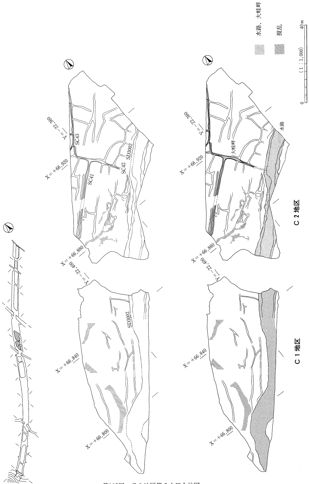
第105図 C2地区第6水田全体図
