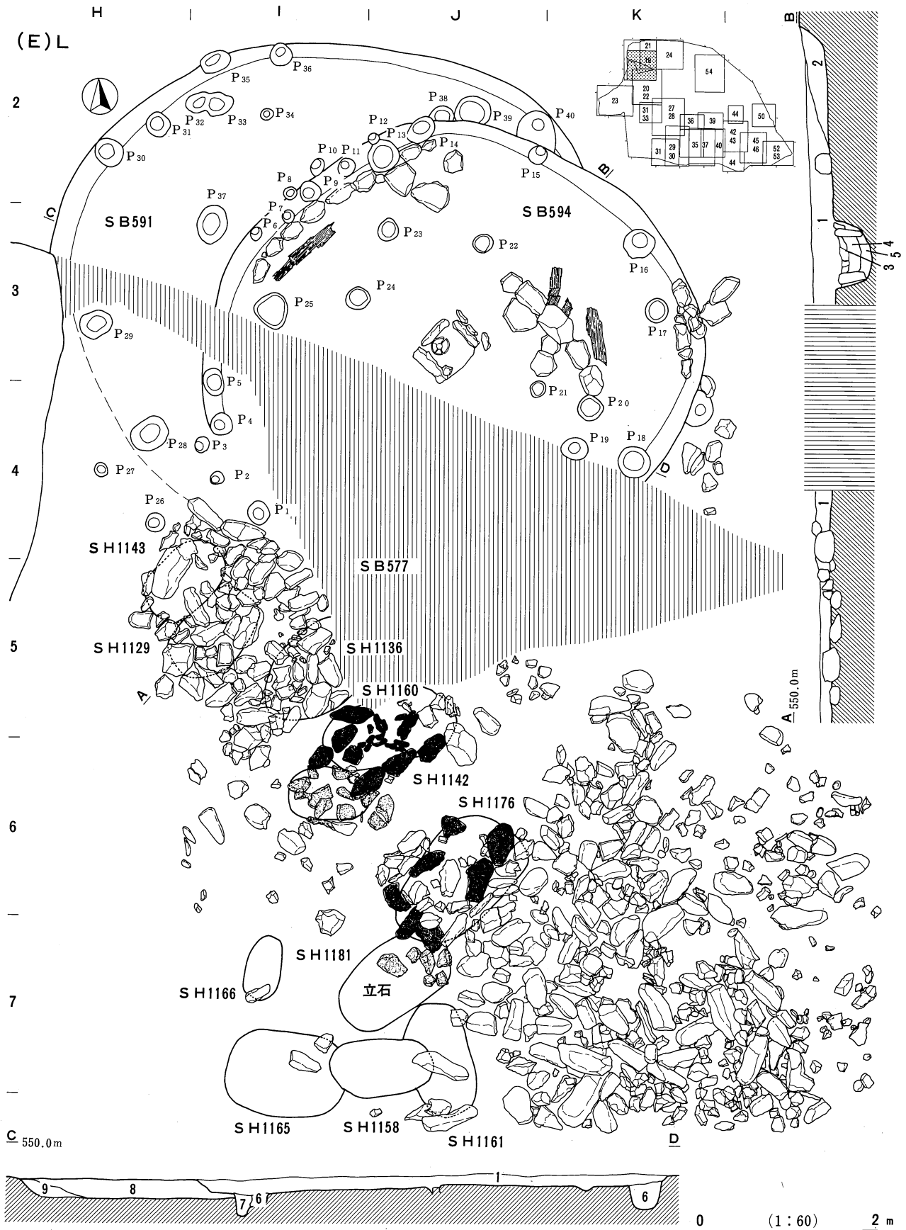
図版19 縄文遺構図9 (S B577・591・594, S H1129ほか) (1:60)
