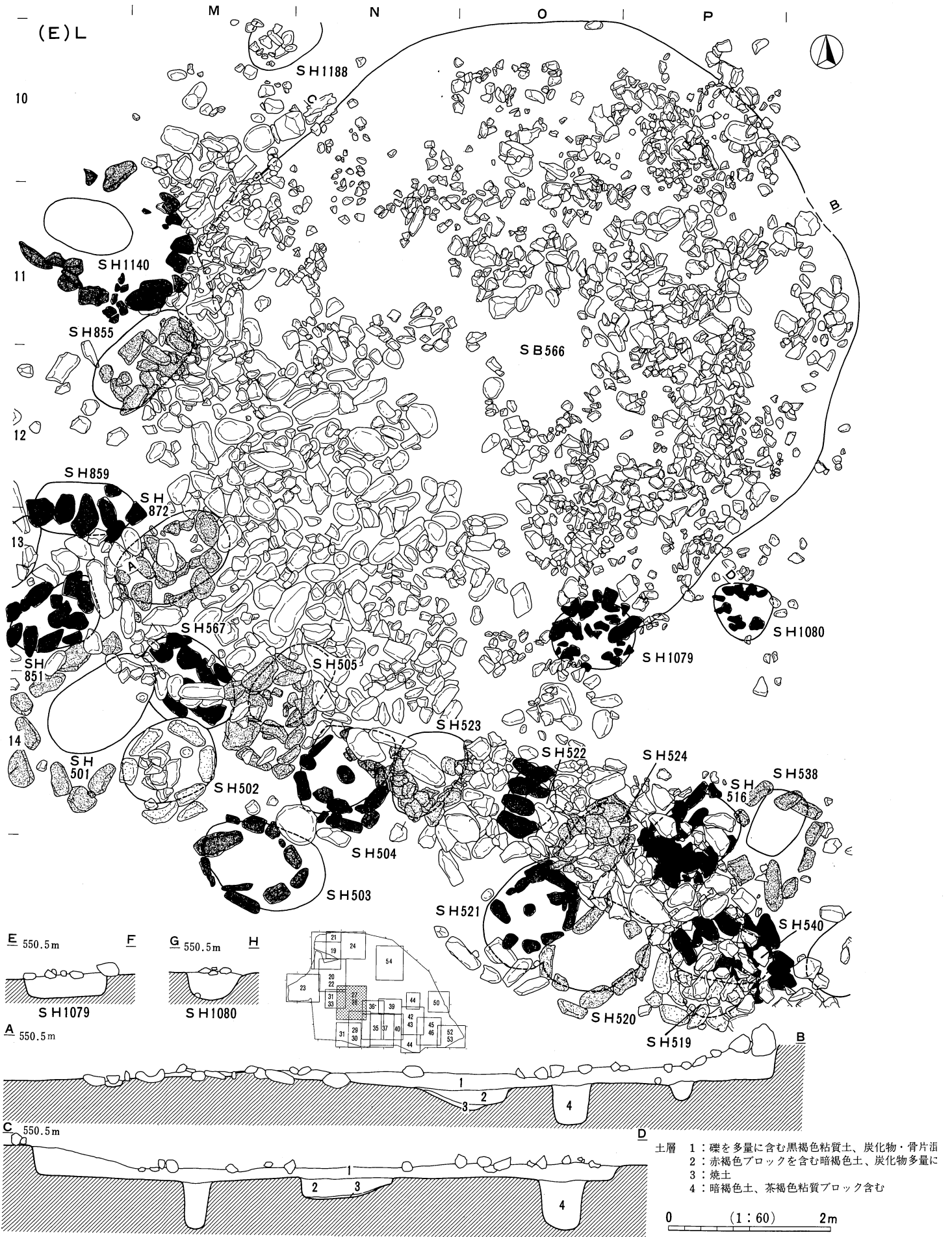
図版27 縄文遺構図17 (S B566, S H501ほか)
