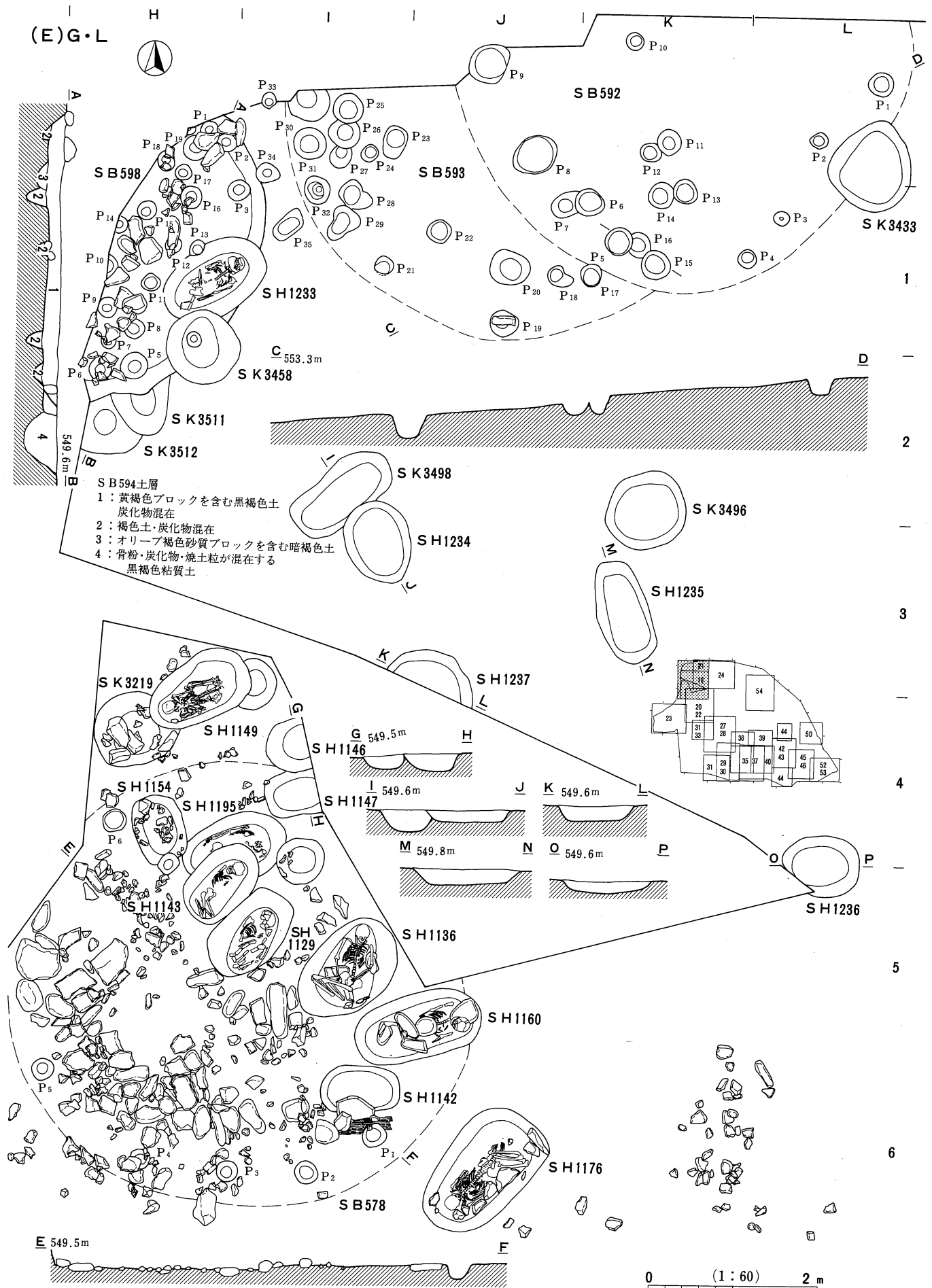
図版21 縄文遺構図11 (S B578・592・593・598, S H1129ほか, S K3219ほか)
