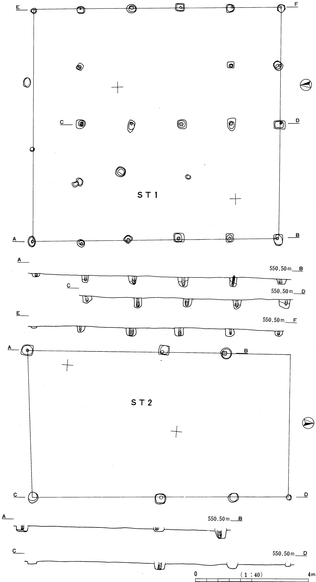
図版59 古代遺構図4 (ST1・2)
